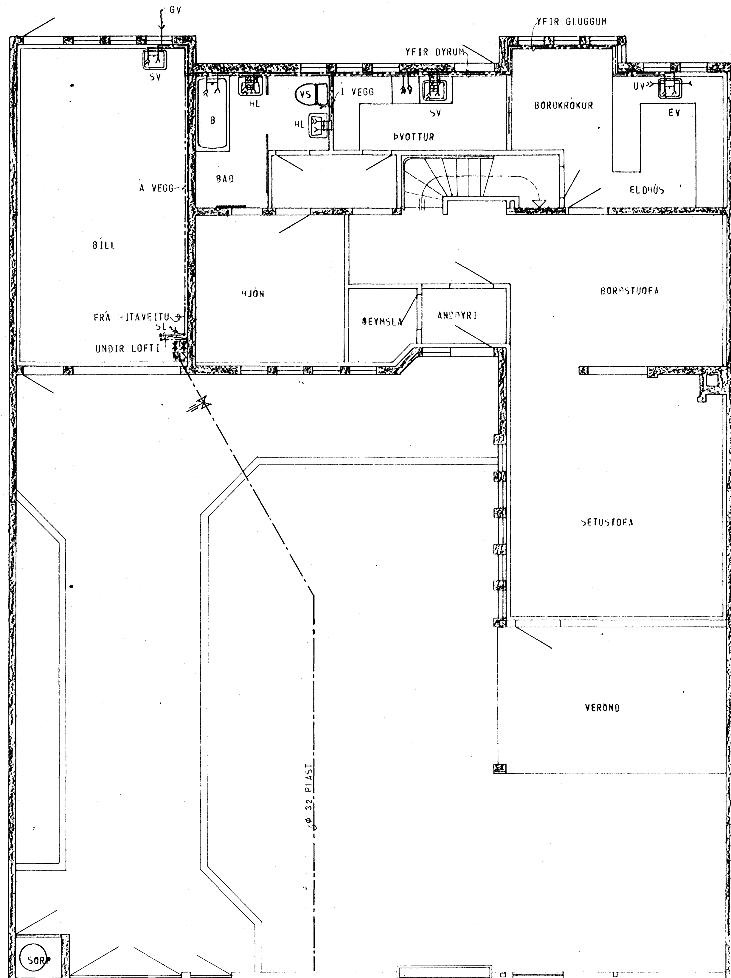
GRUNNMYND - HÆÐAR 1:50
