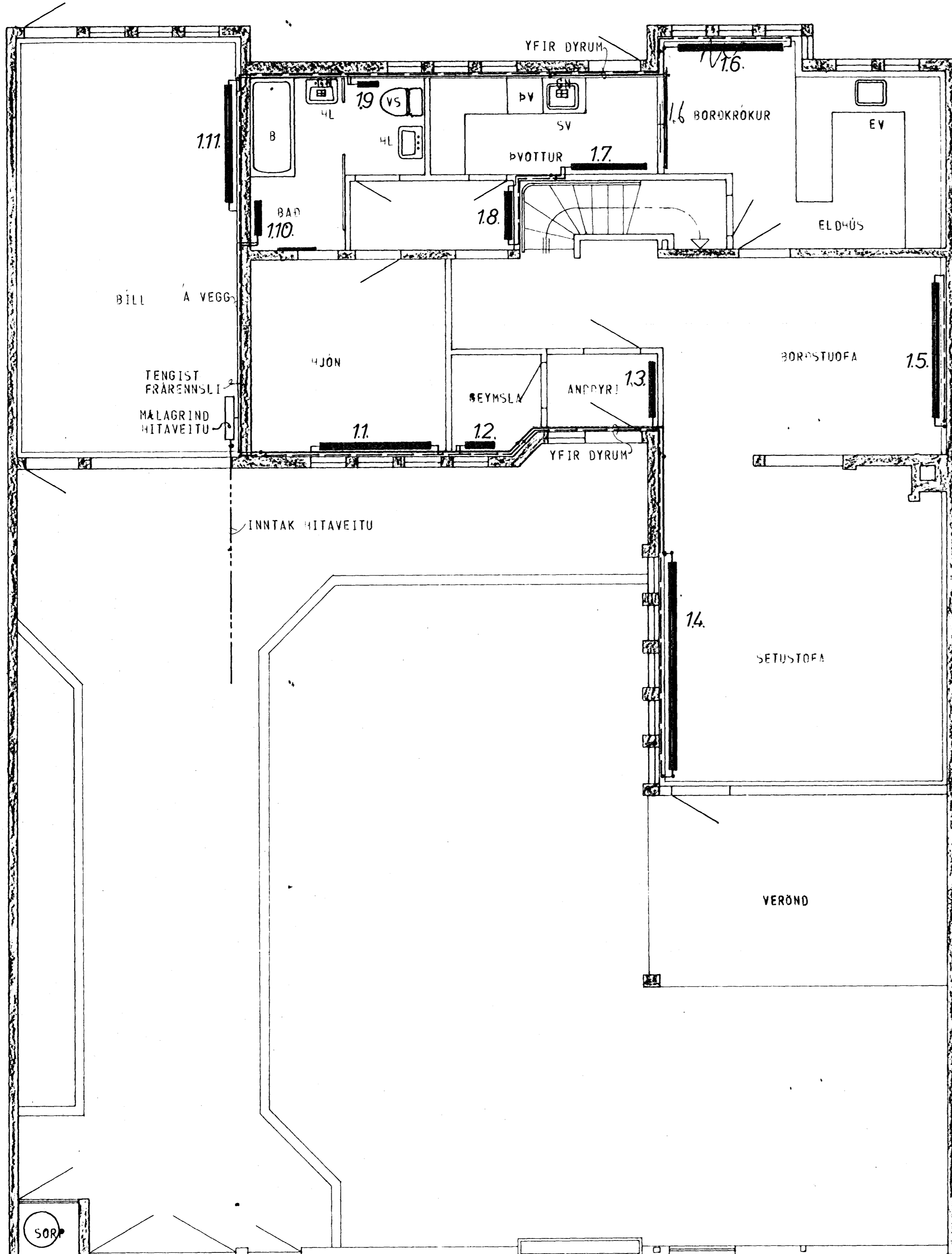
GRUNNMYND - HÆÐAR 1:50
