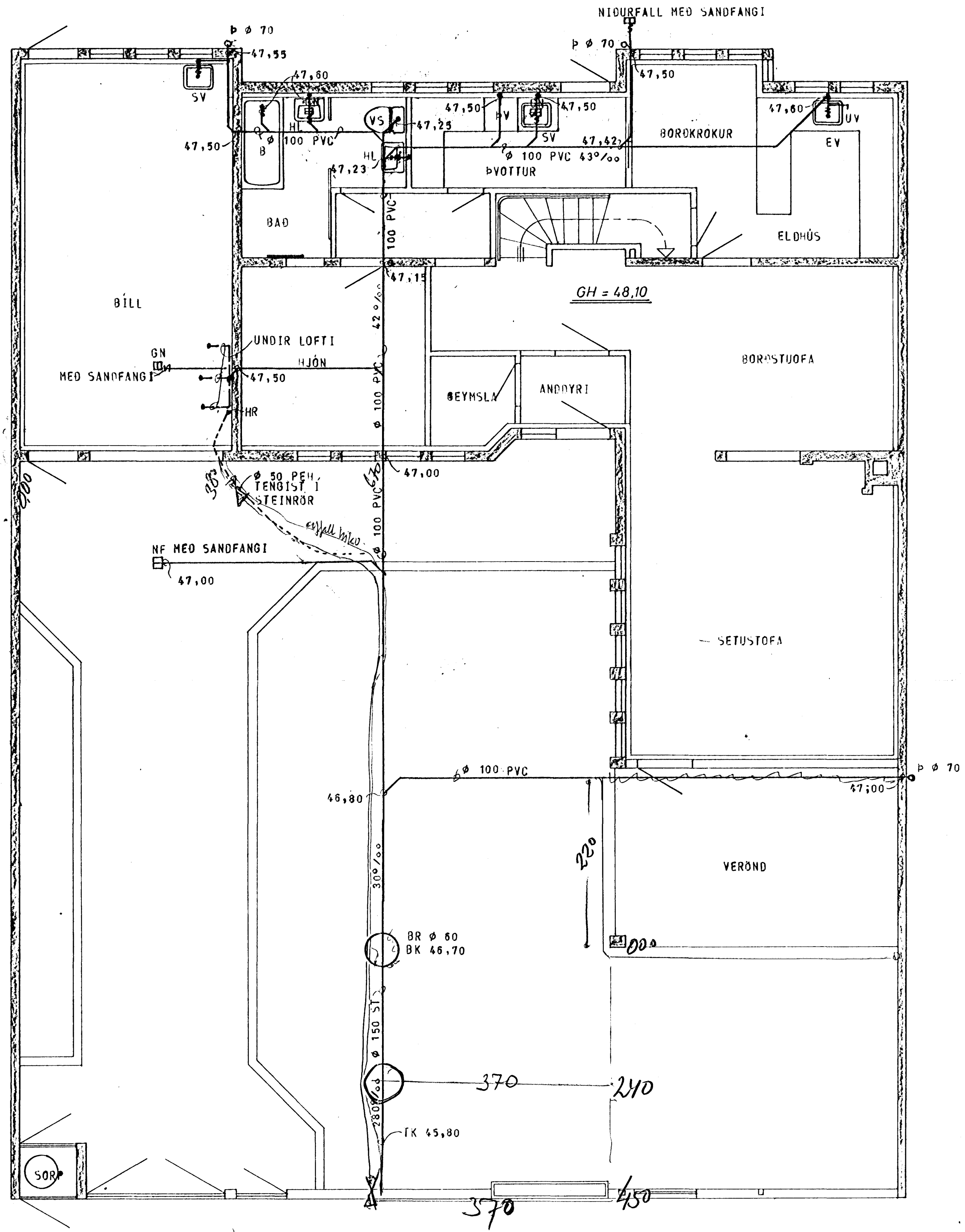
GRUNNMYND - HÆÐAR 1:50
