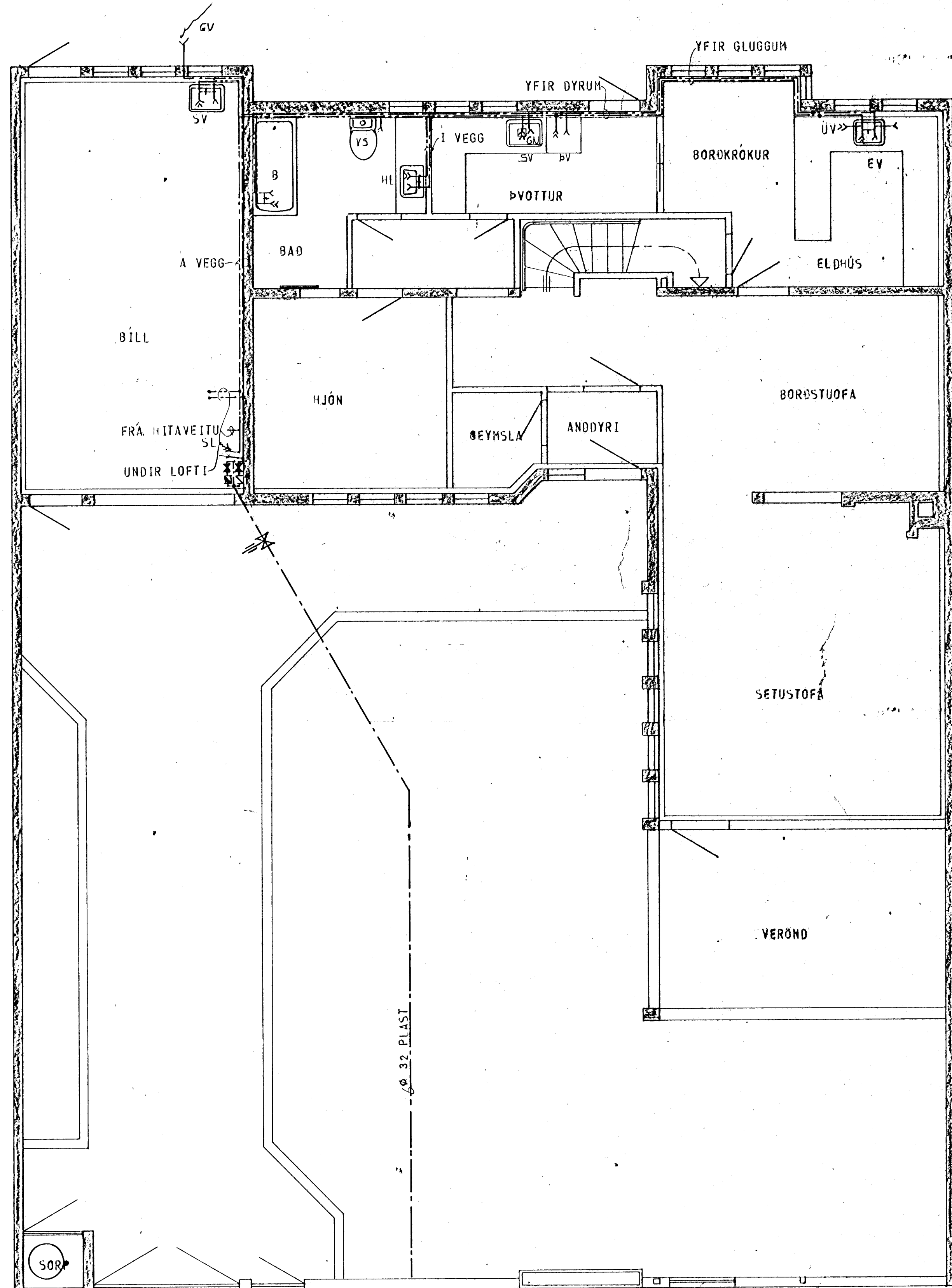
GRUNNMYND - HÆÐAR 1:50
