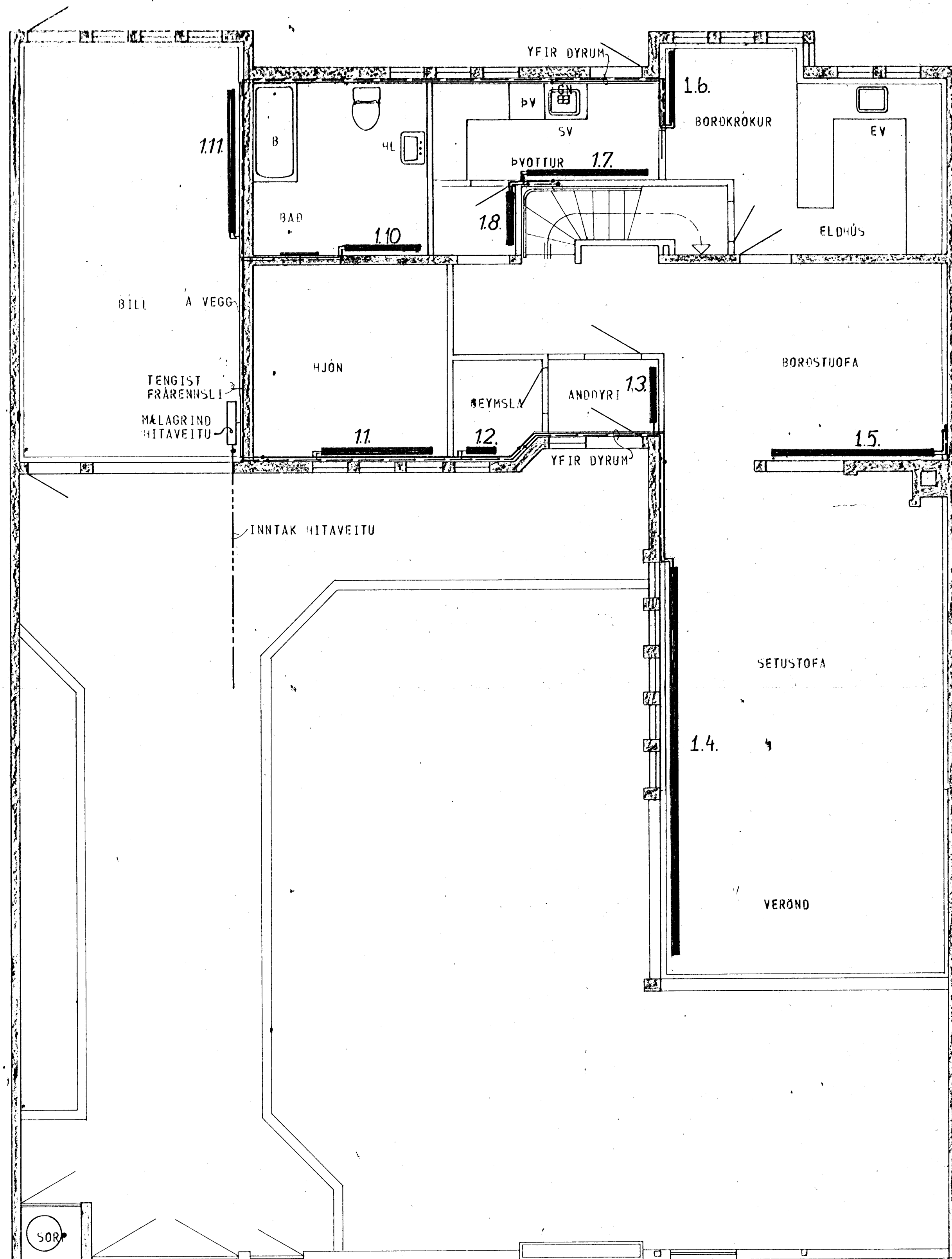
GRUNNMYND - HÆÐAR 1:50
