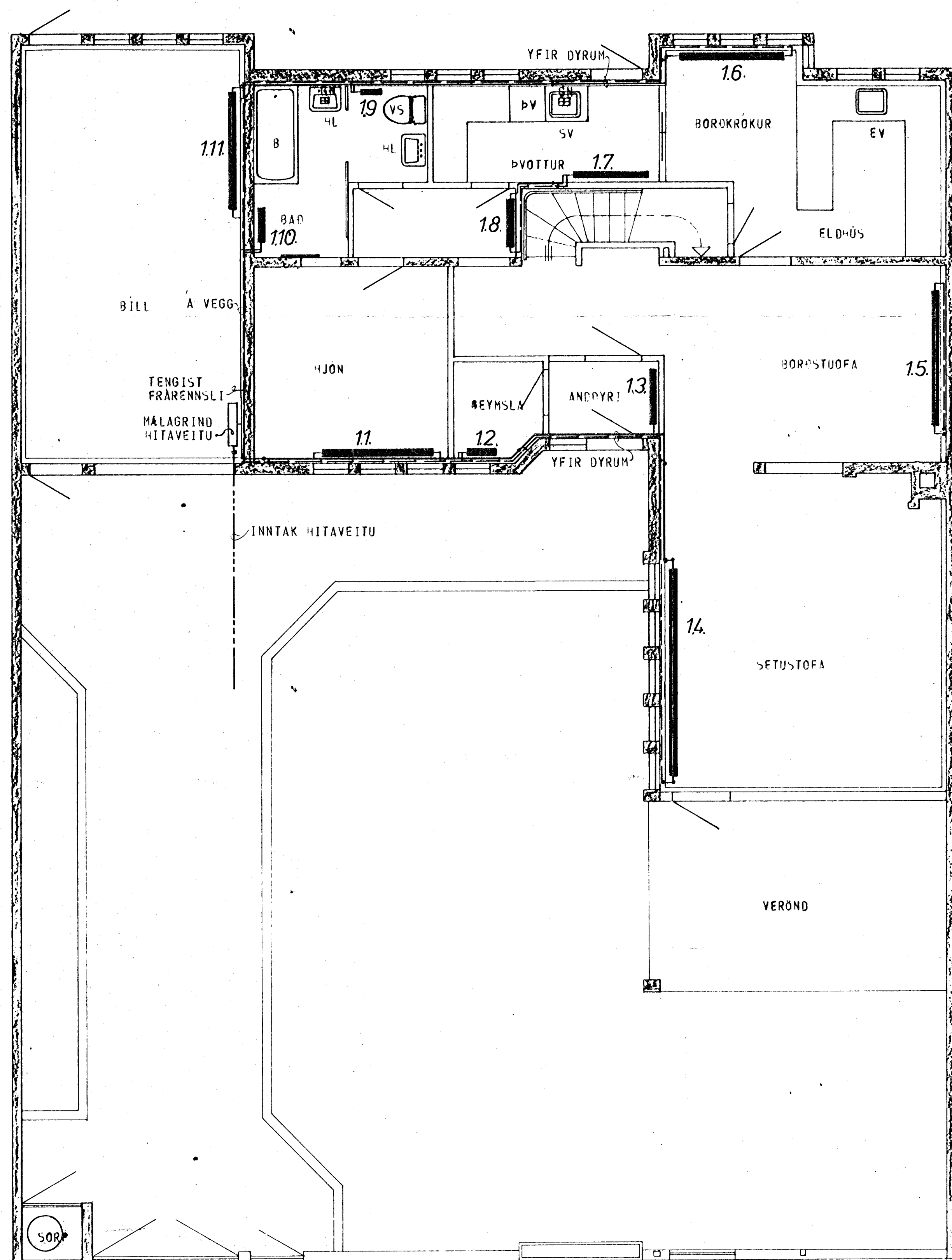
GRUNNMYND - HÆÐAR 1:50
