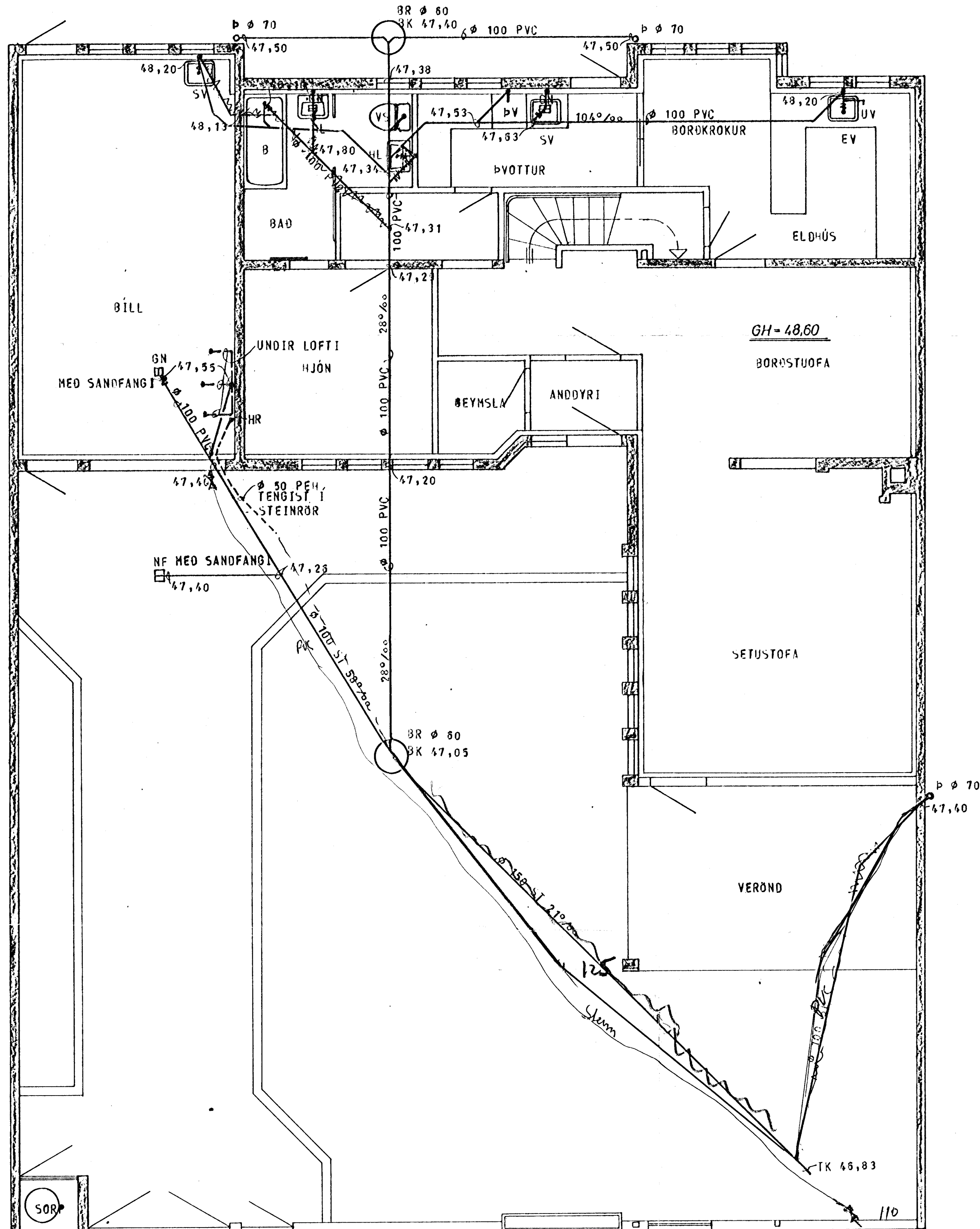
GRUNNMYND - HÆÐAR 1:50
