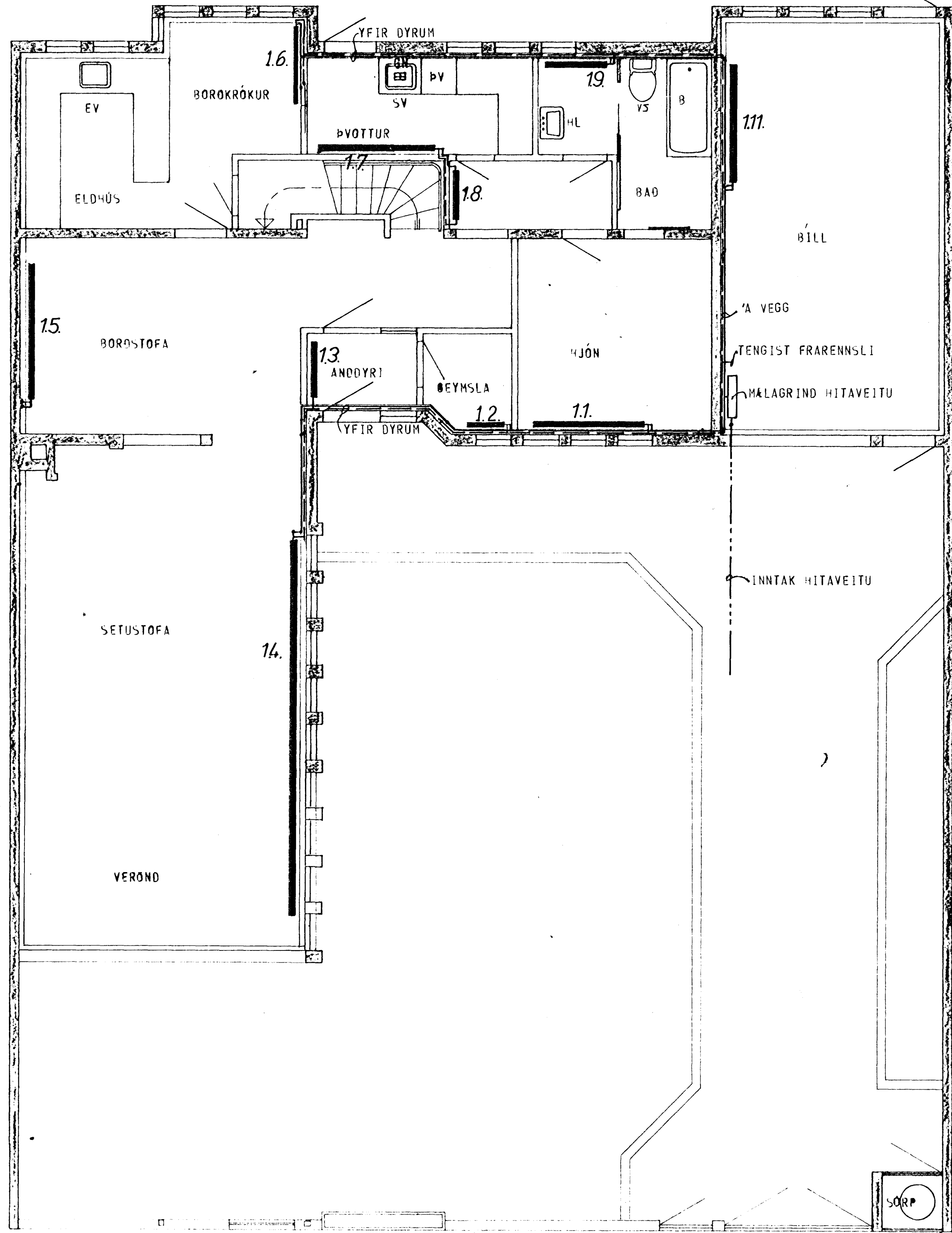
GRUNNMYND - HÆÐAR 1:50
