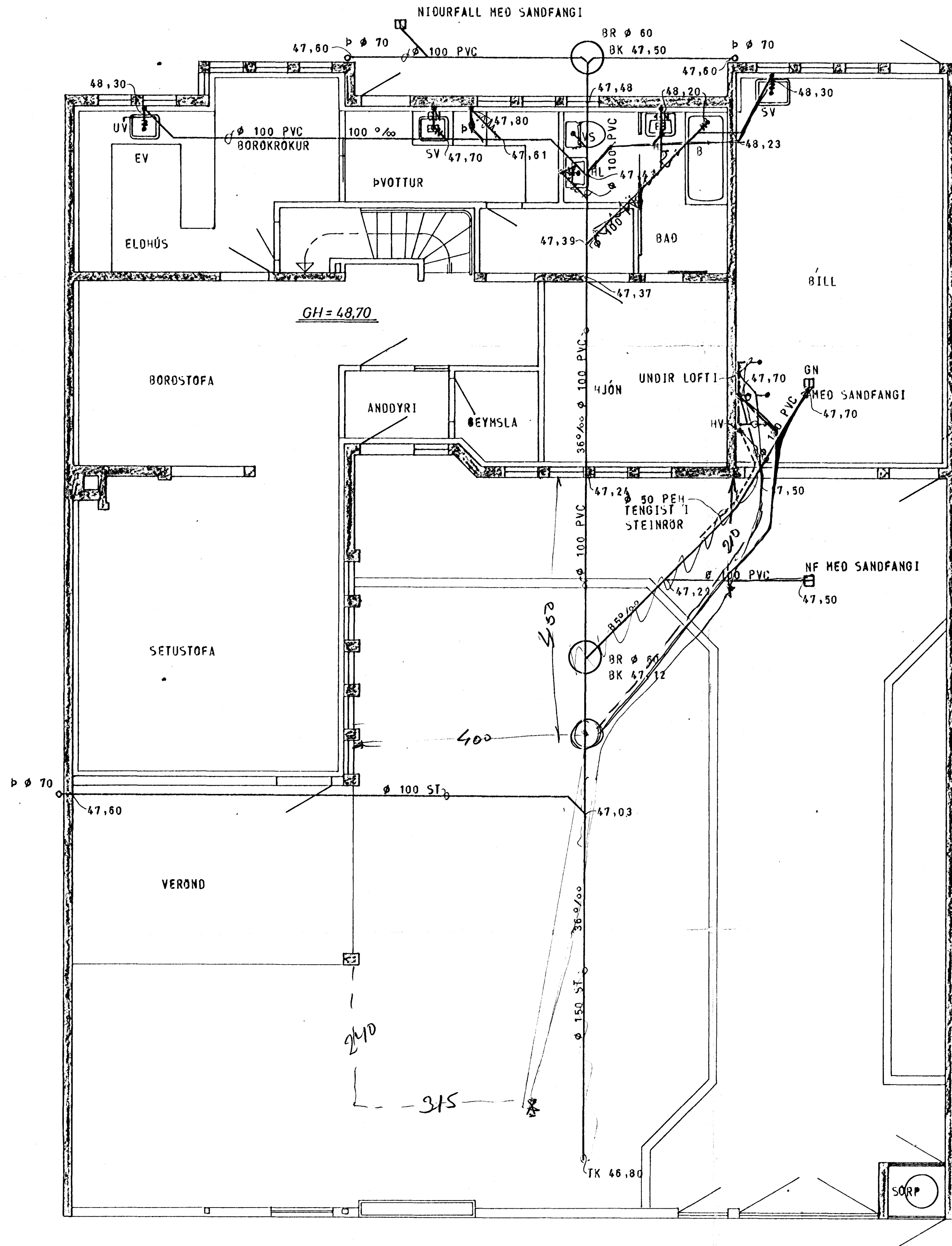
GRUNNMYND - HÆÐAR 1:50
