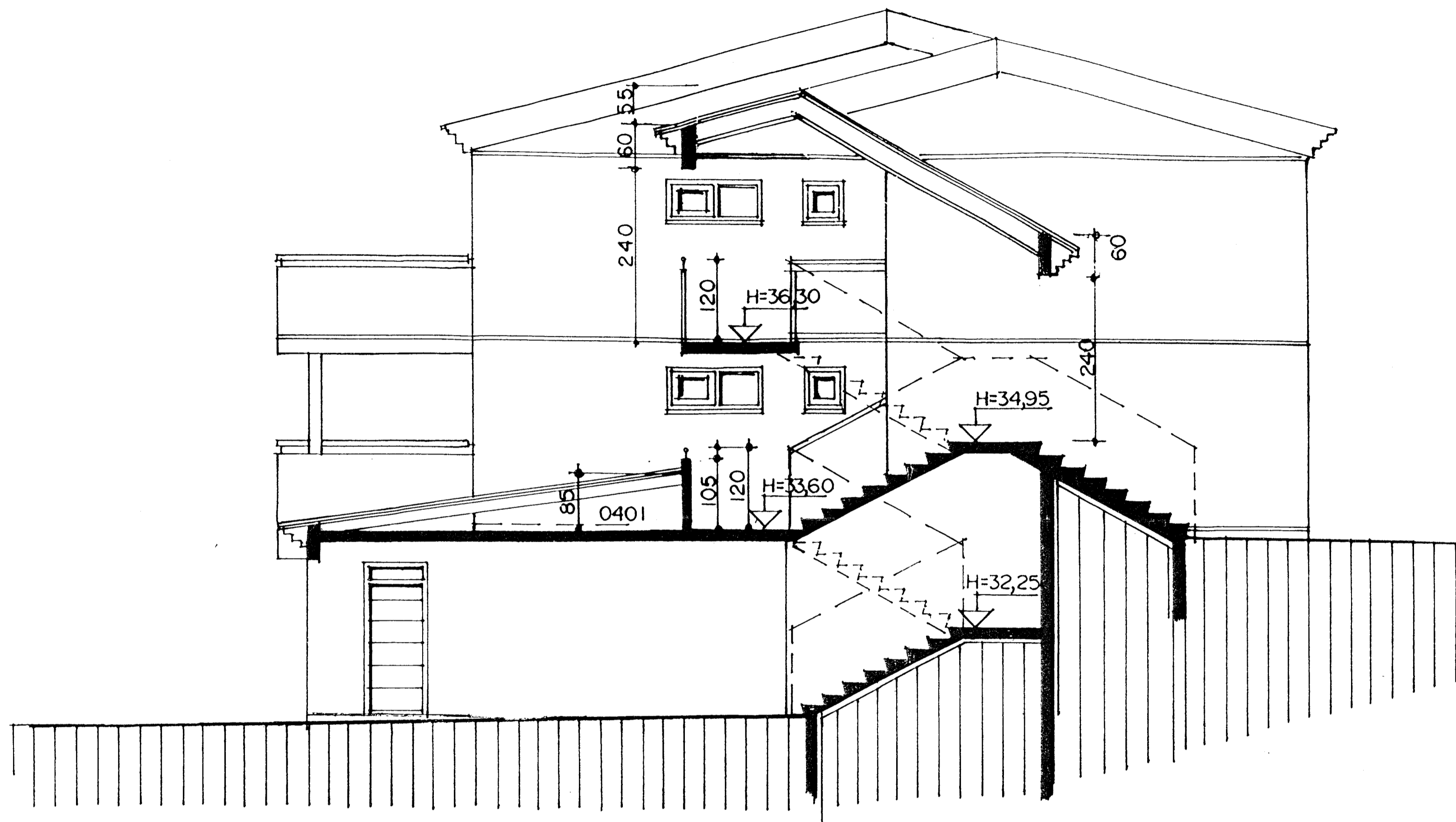
SNÍÐ A-A MKV. 1:50.
