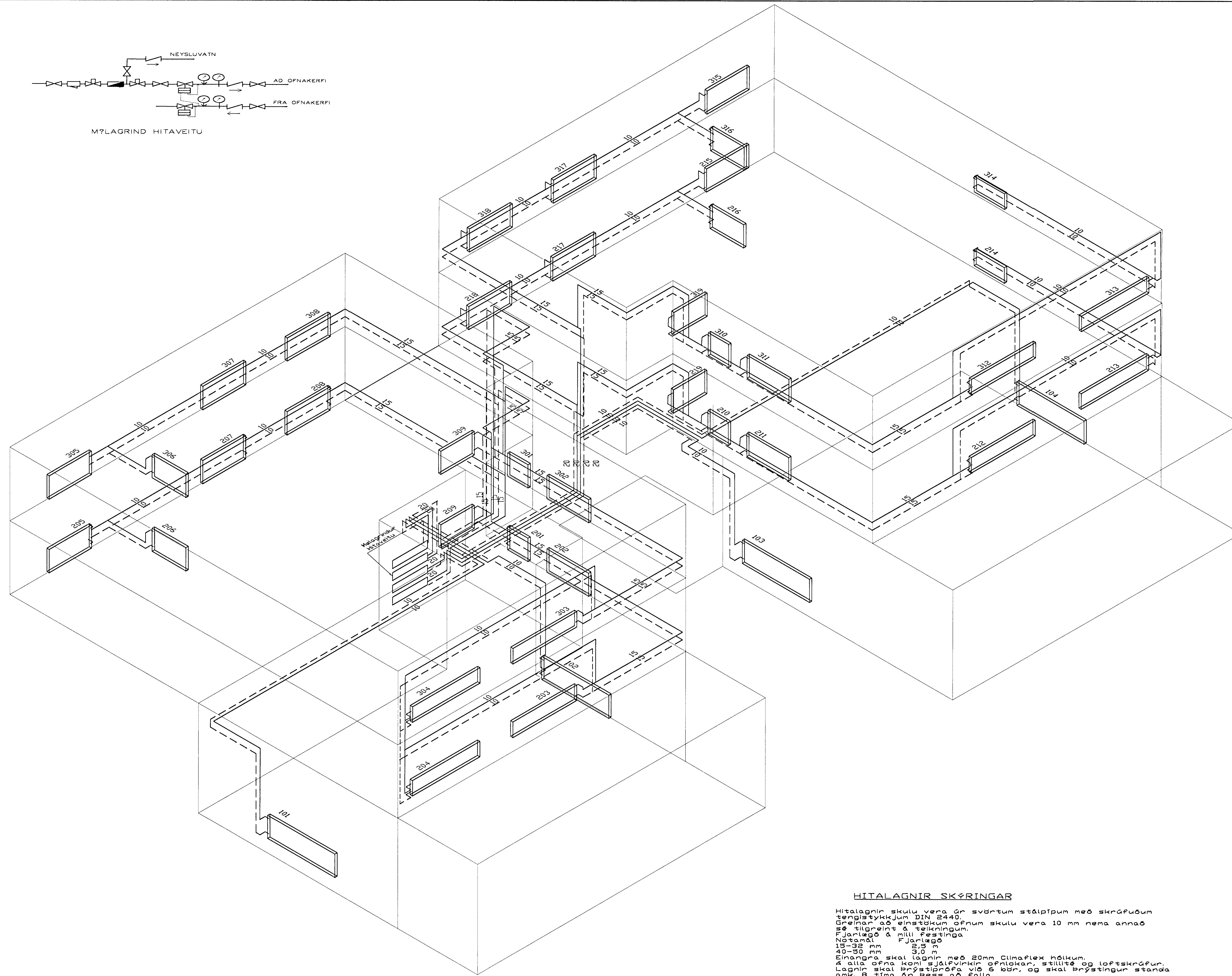
Hitlagnir, rúmmynd, 1:50
