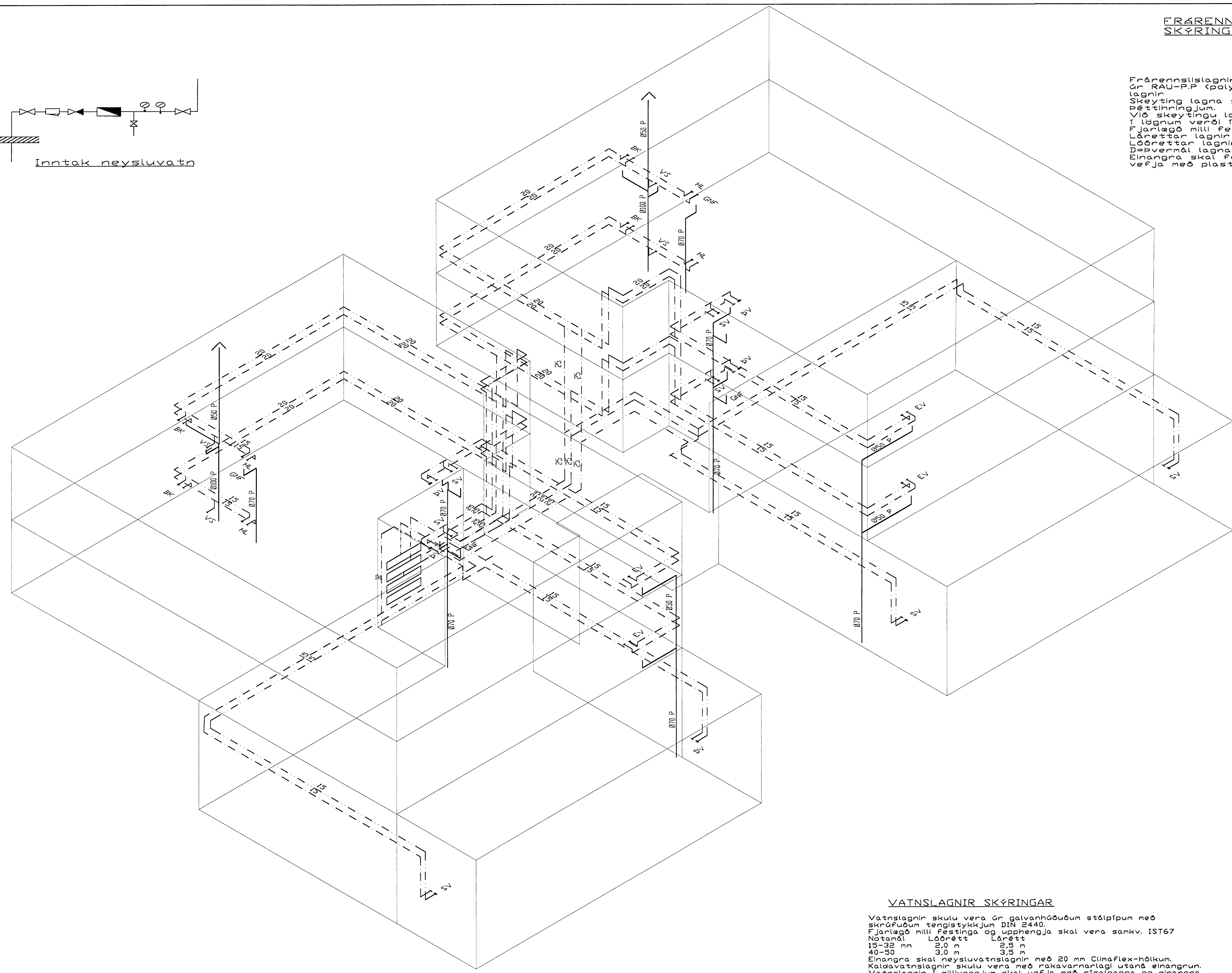
Vatnslagnir, rúmmýnd, 1:50
