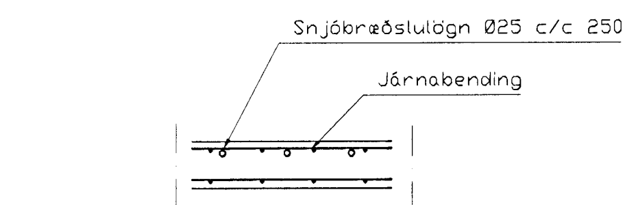
Snjóbræðsla snið, 1:20
