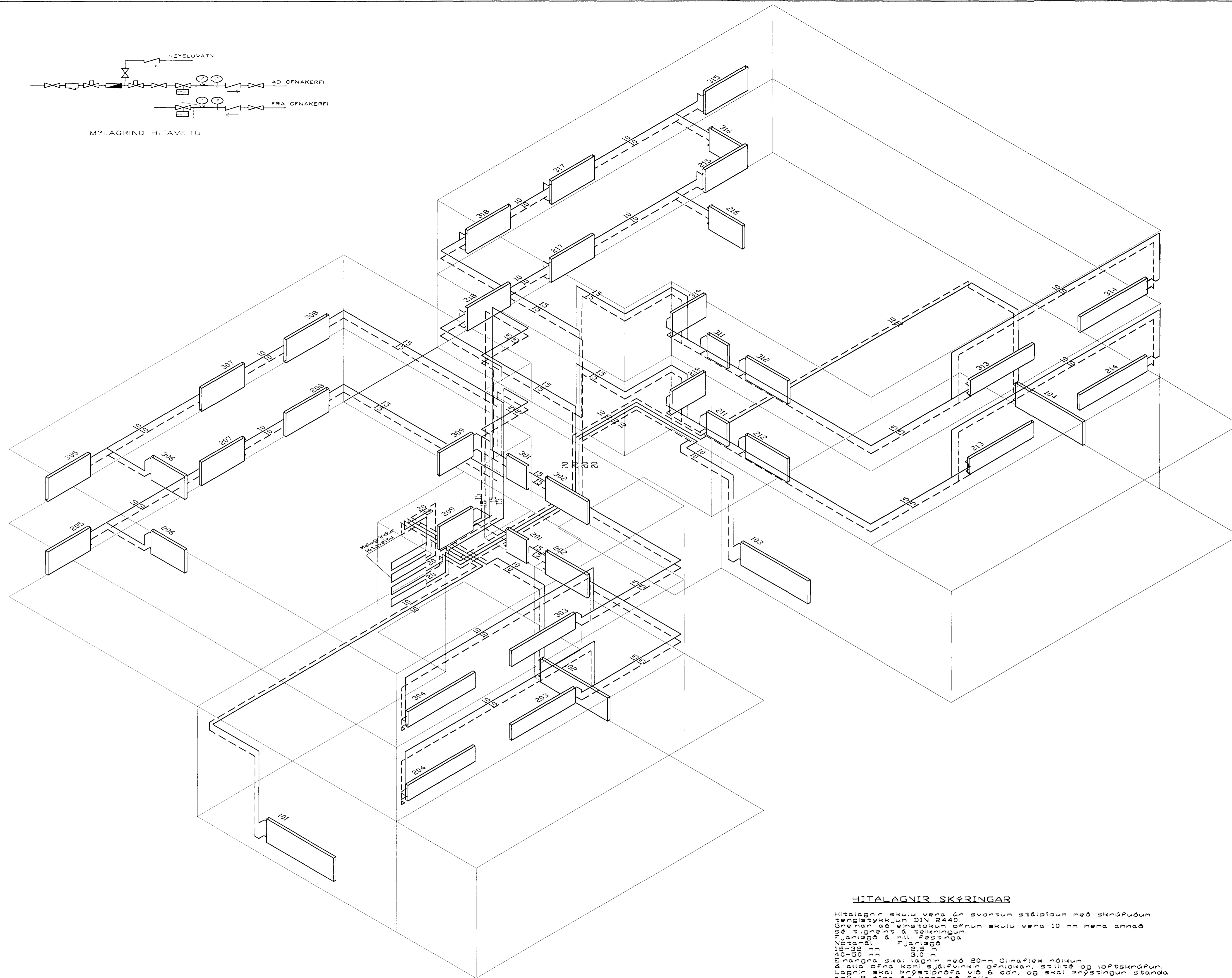
Hitalagnir, rúmmynd, 1:50
