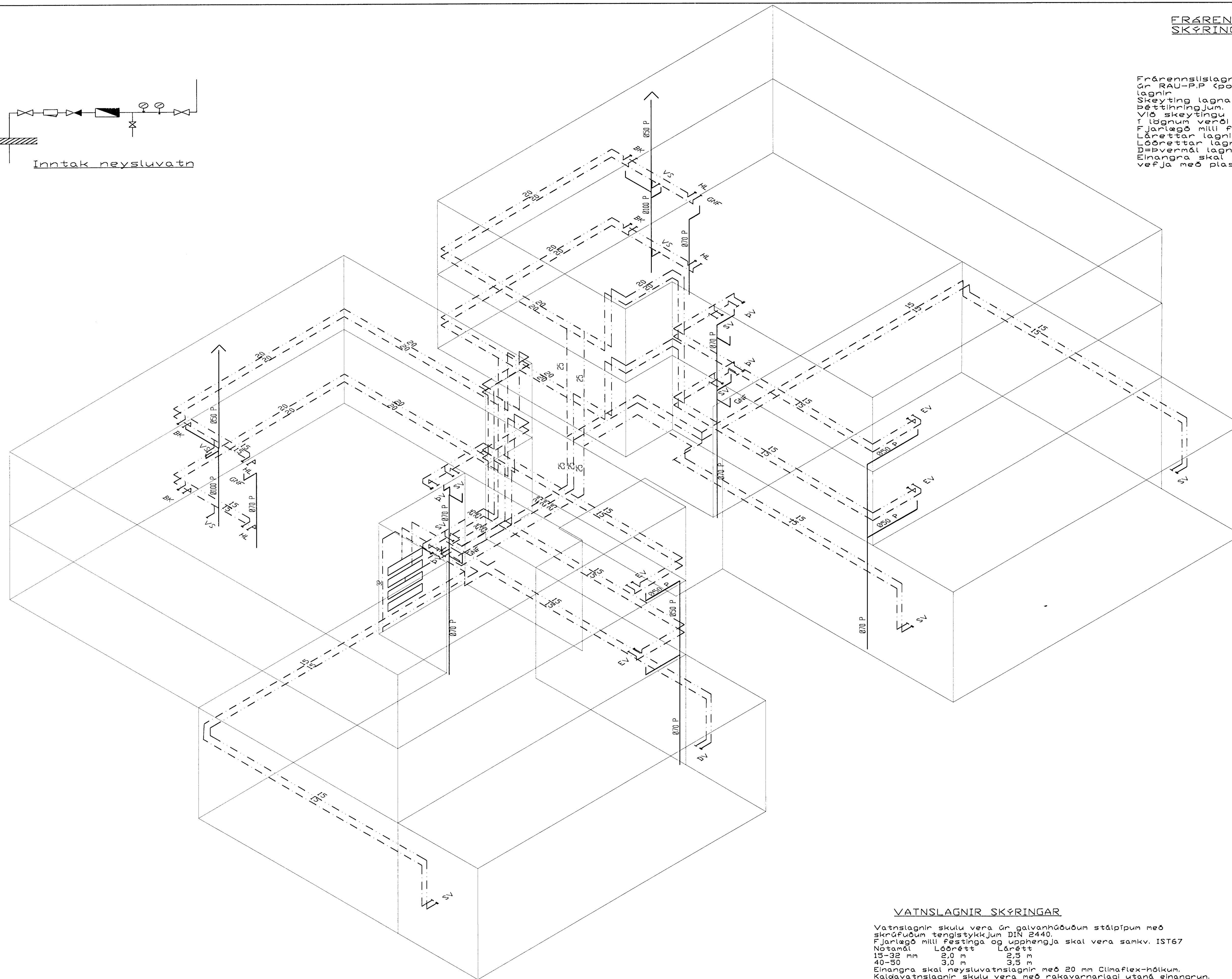
Vatnslagnir, rúmynd, 1:50
