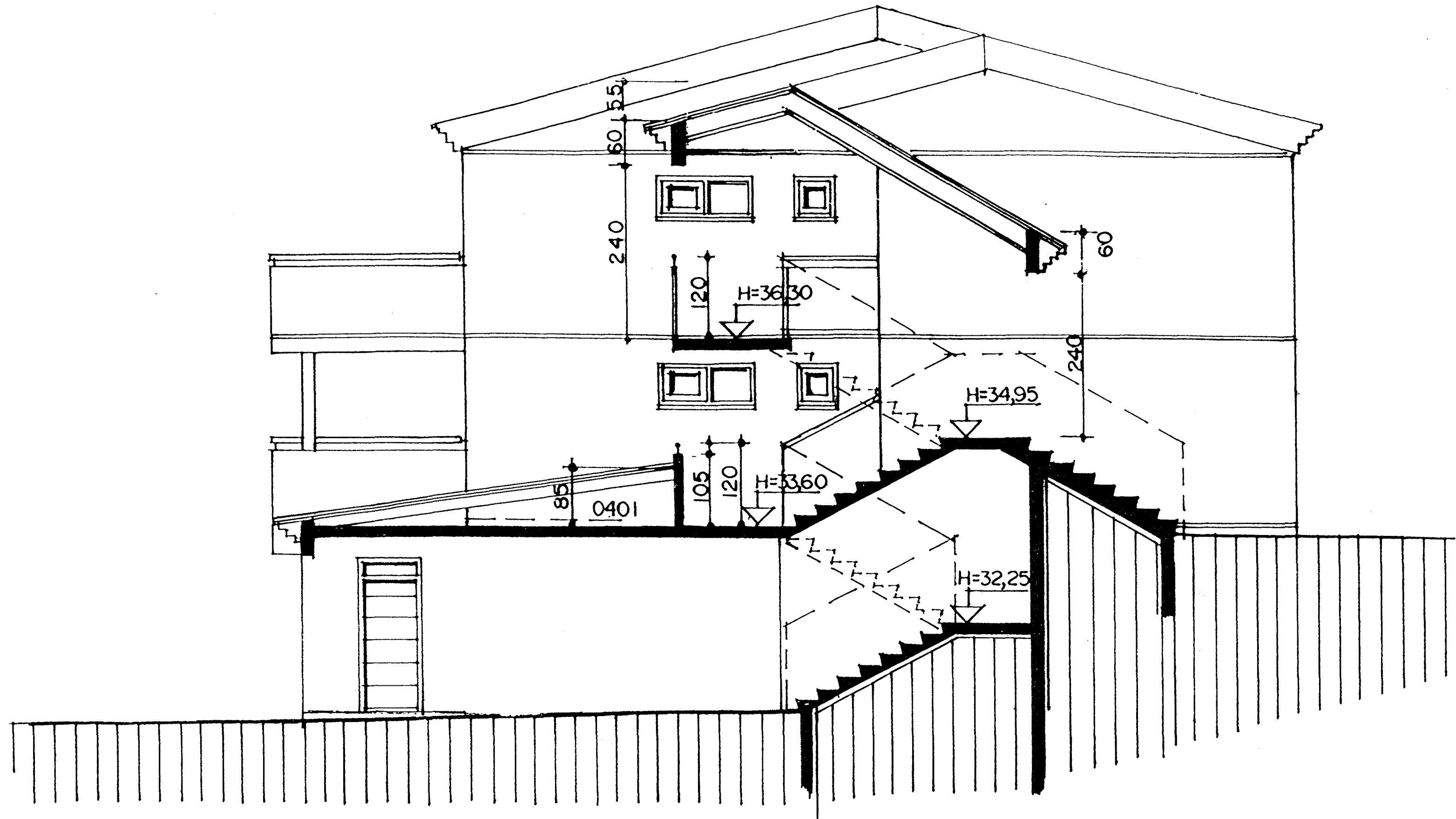
SNID A-A MKV. 1:50.
