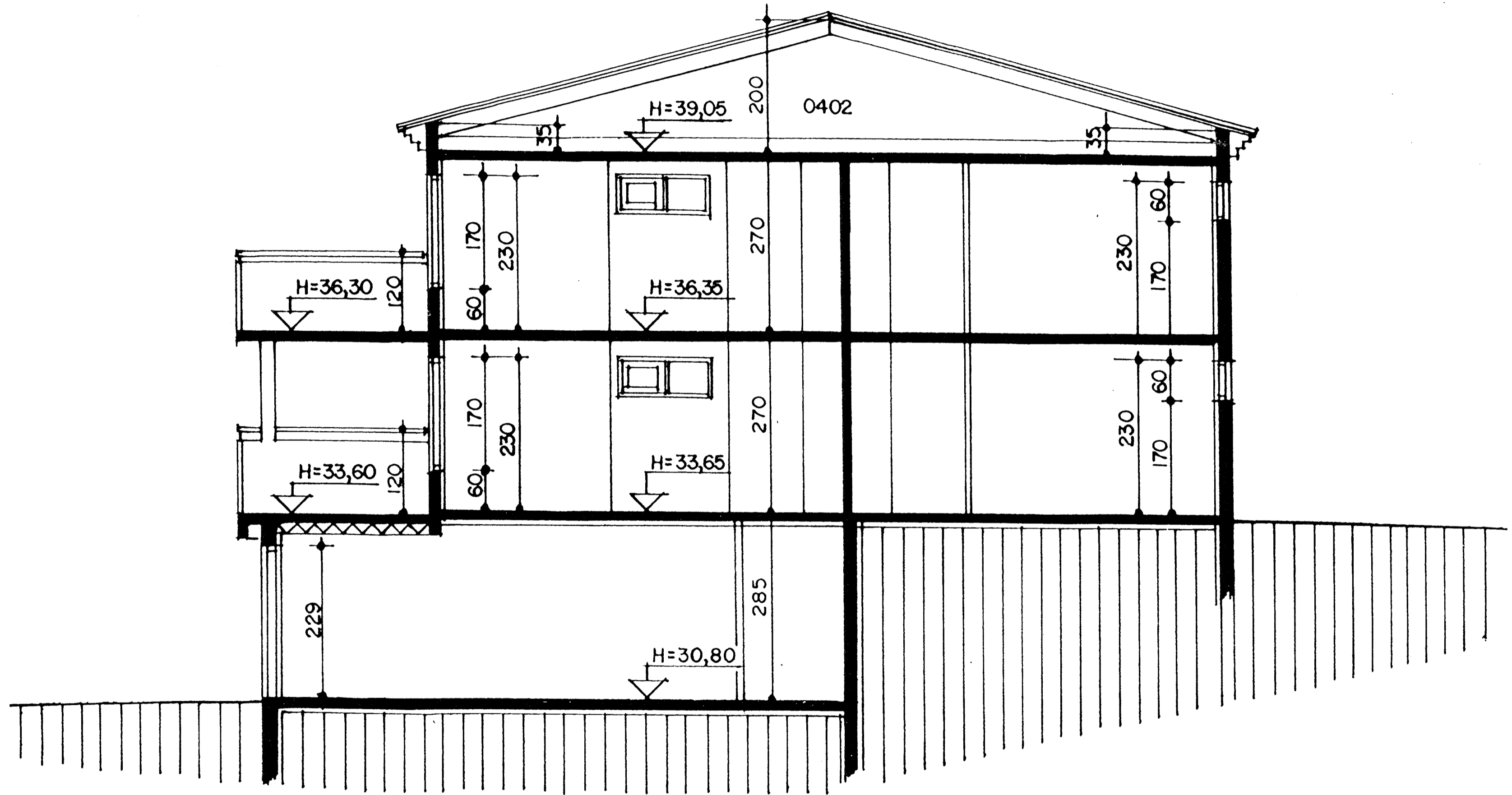
SNÍÐ B-B MKV. 1:50.
