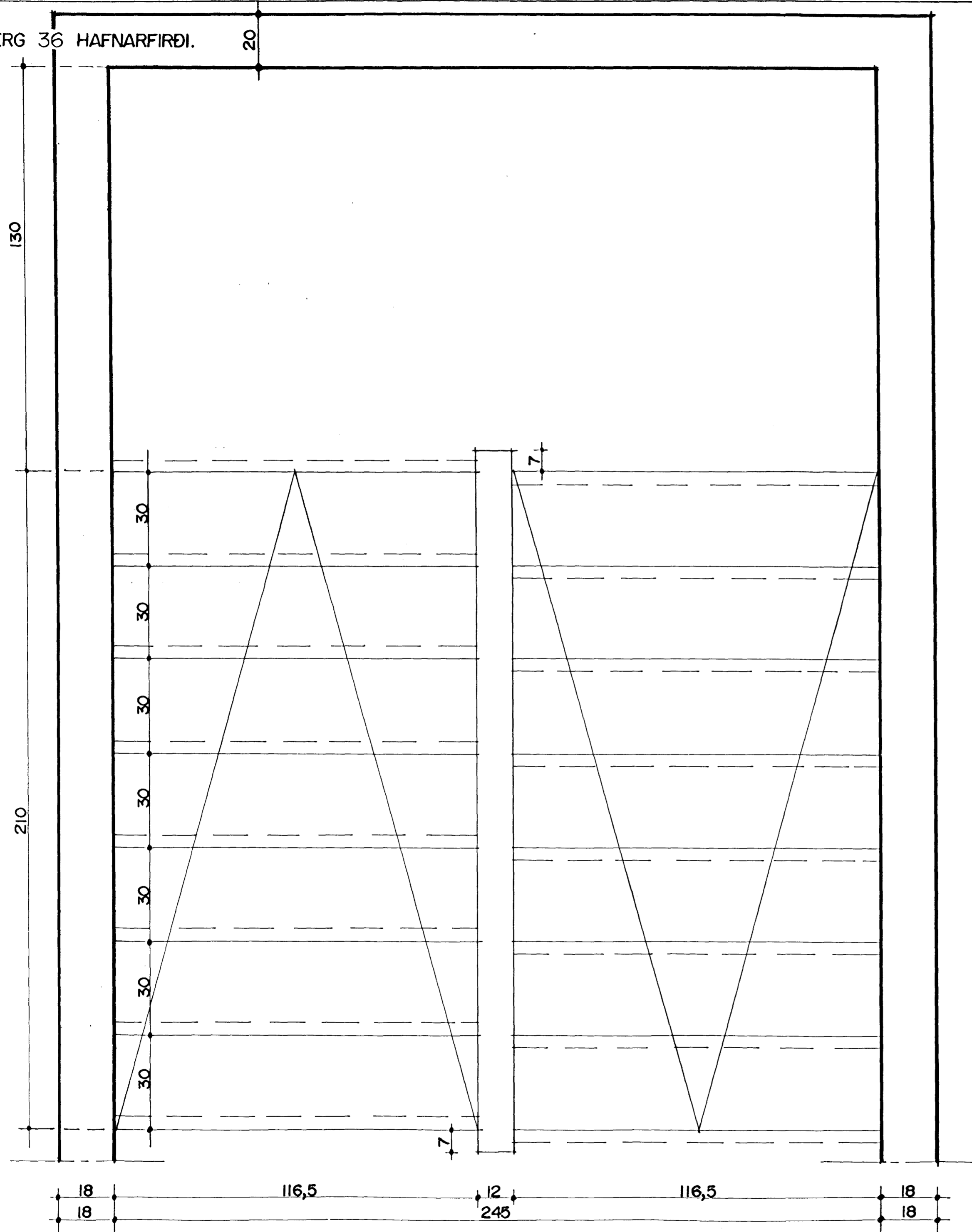
GRUNNMYND STIGI MKV. 1:10.
