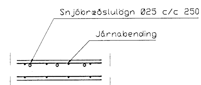
Snjóbræðsla snið, 1:20
