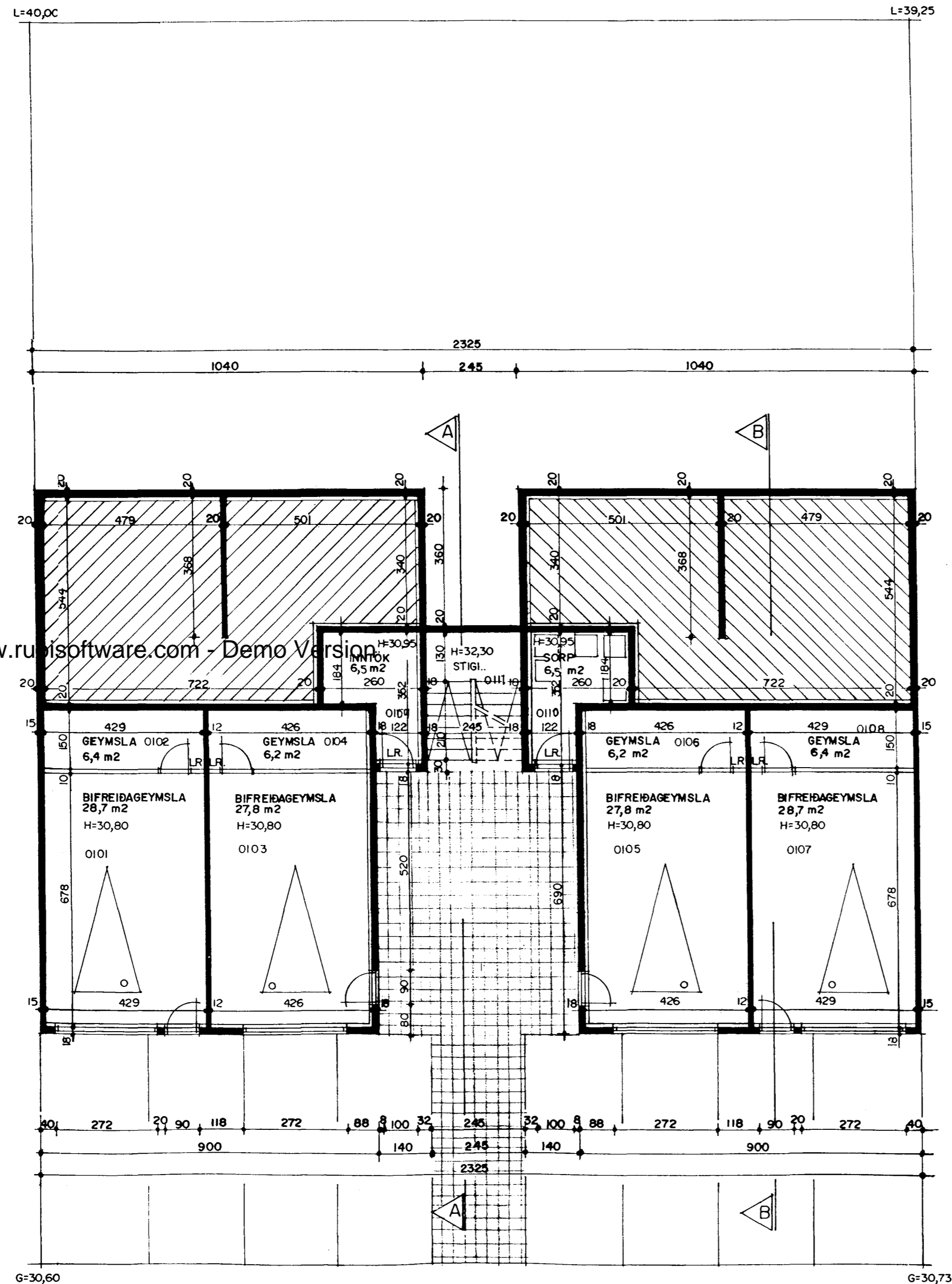
G=30,60 GRUNNMYND I HÆÐ/JARÐHÆÐ MKV. 1:100. G=30,73
