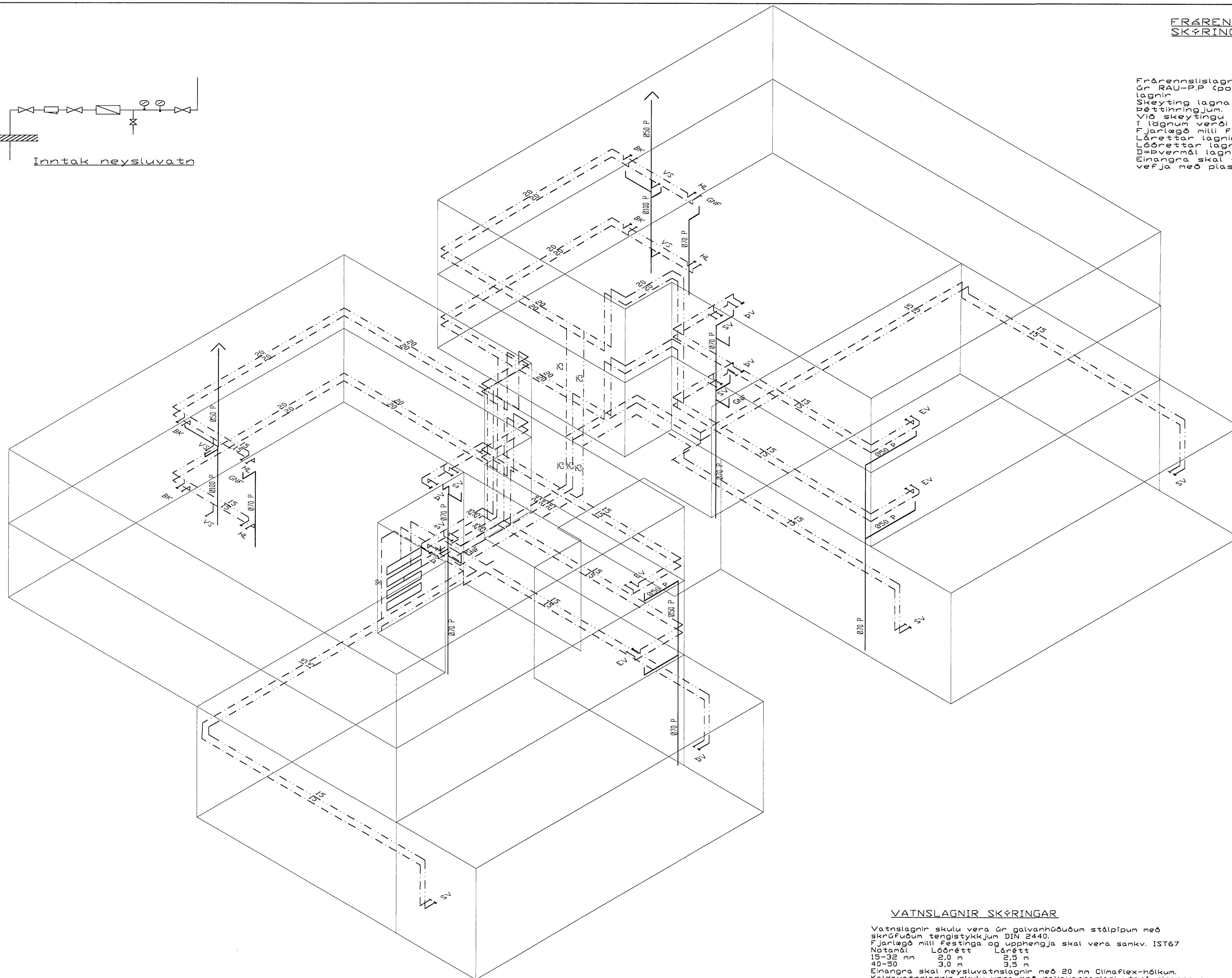
Vatnslagnir, rúmynd, 1:50
