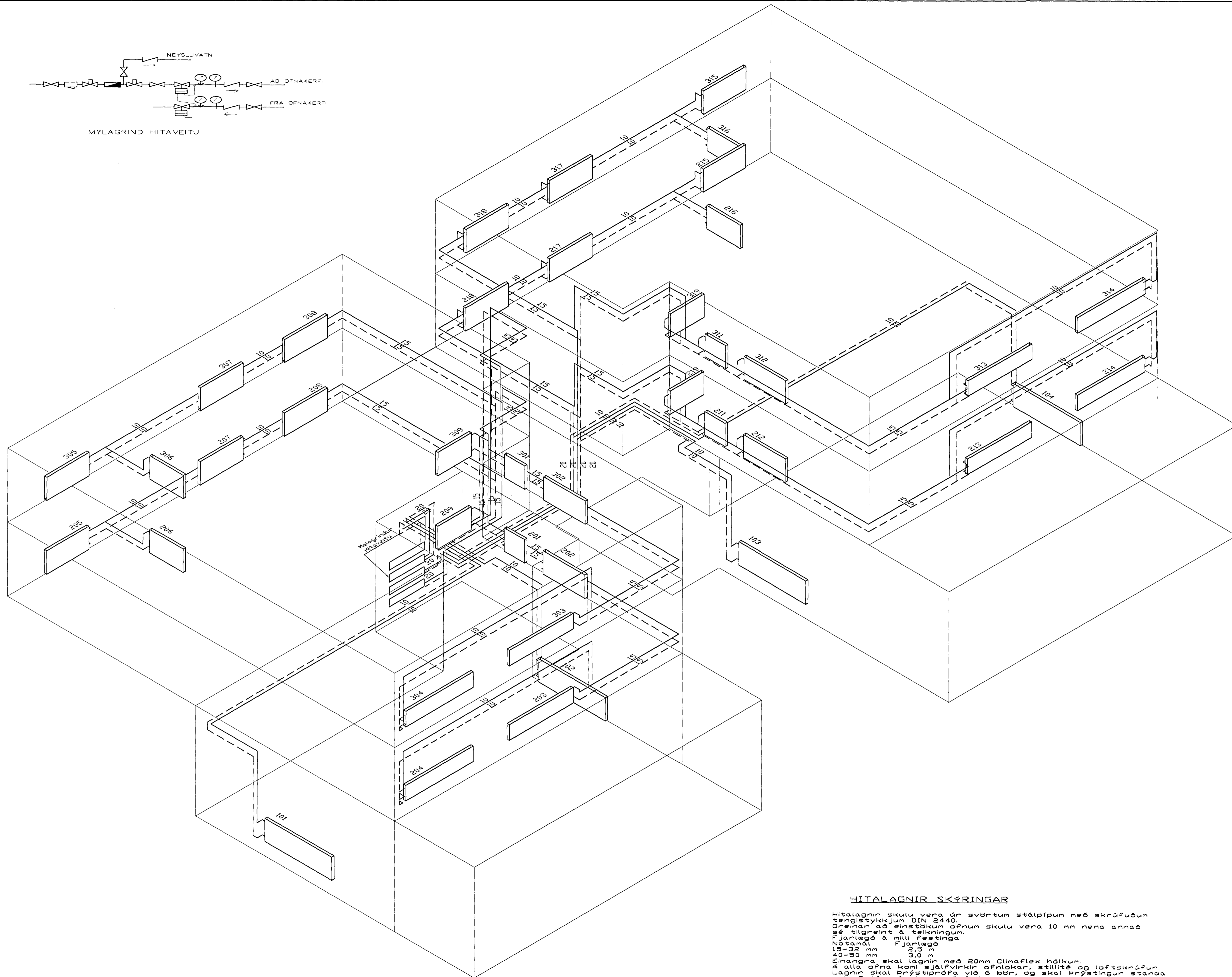
Hitalagnir, rúmynd, 1:50
