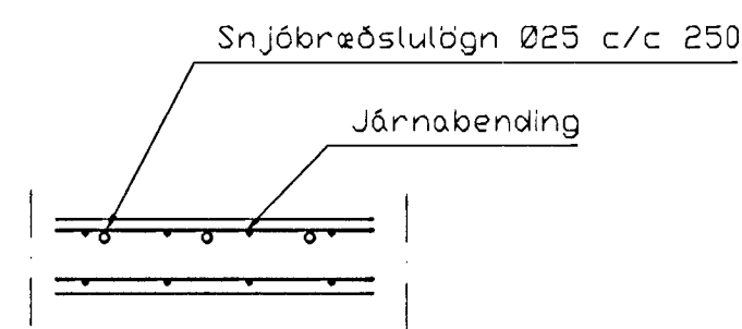
Snjóbræðsla snið, 1:20
