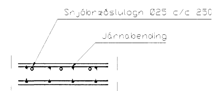
Snjóbræðsla snið, 1:20
