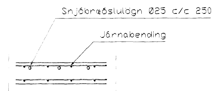
Snjóbræðsla snið, 1:20
