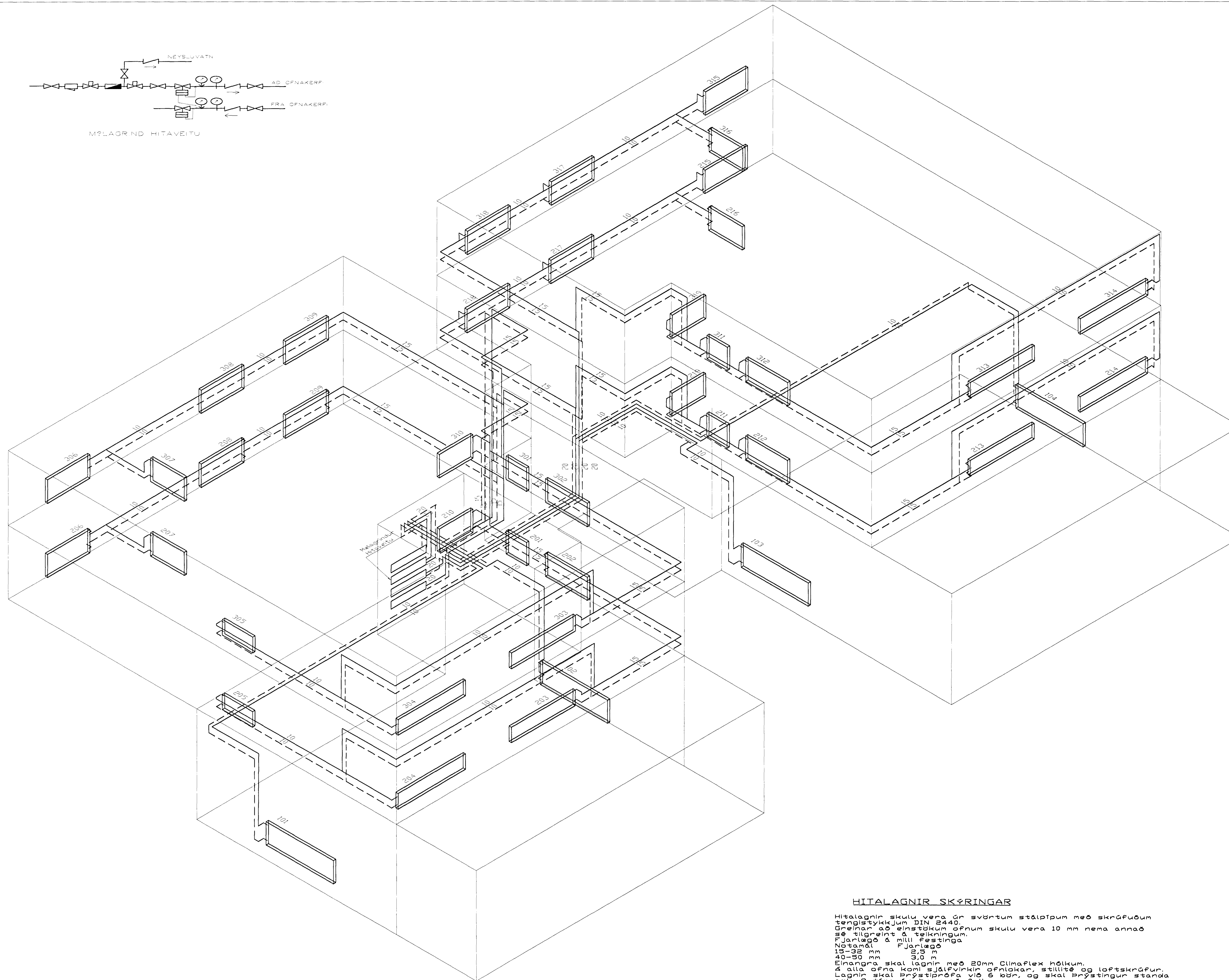
Hitalagnir, rúmmynd, 1:50
