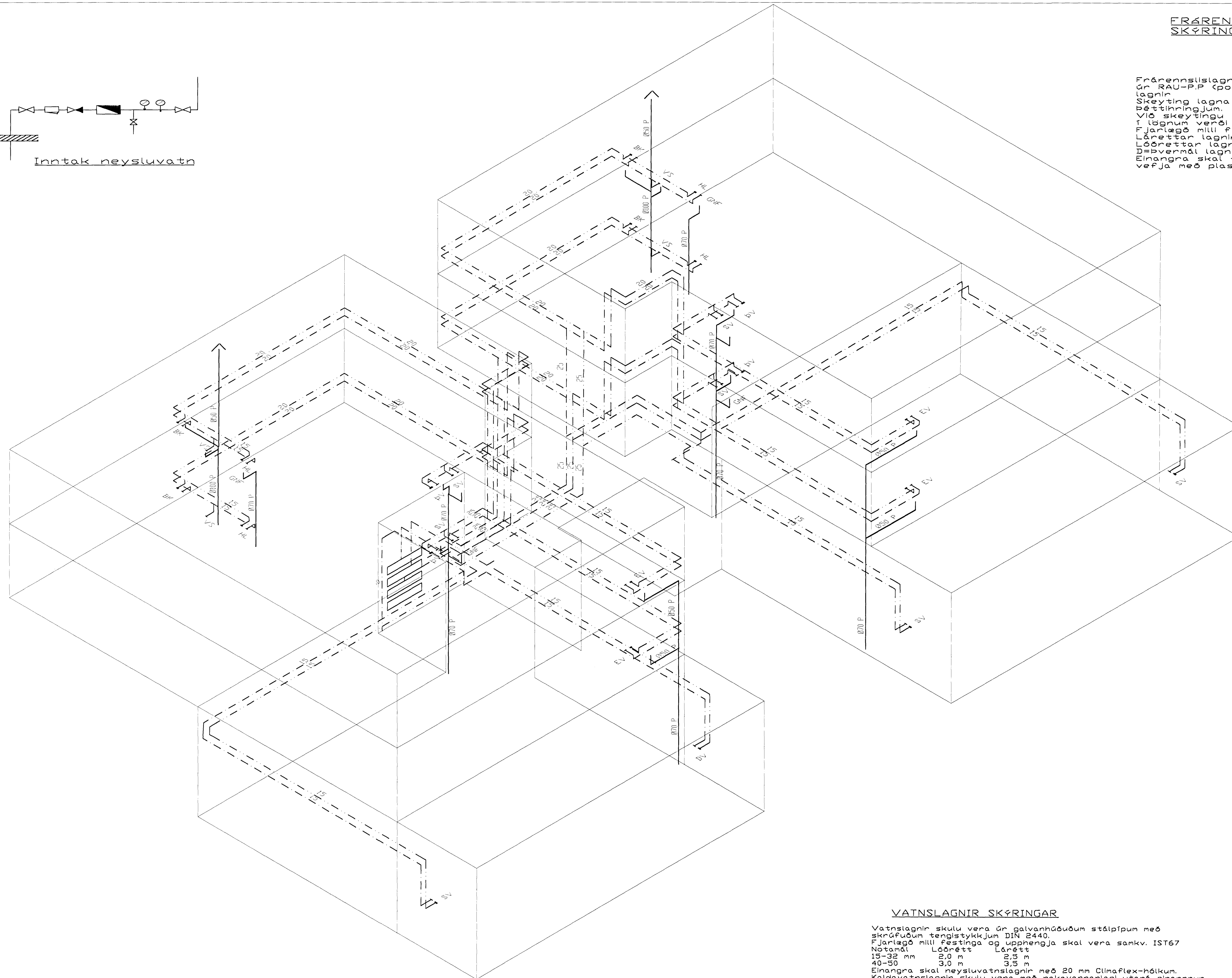
Vatnslagnir, rúmmýnd, 1:50
