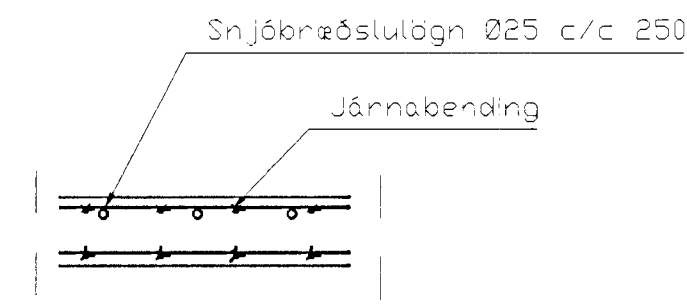
Snjóbræðsla snið, 1:20
