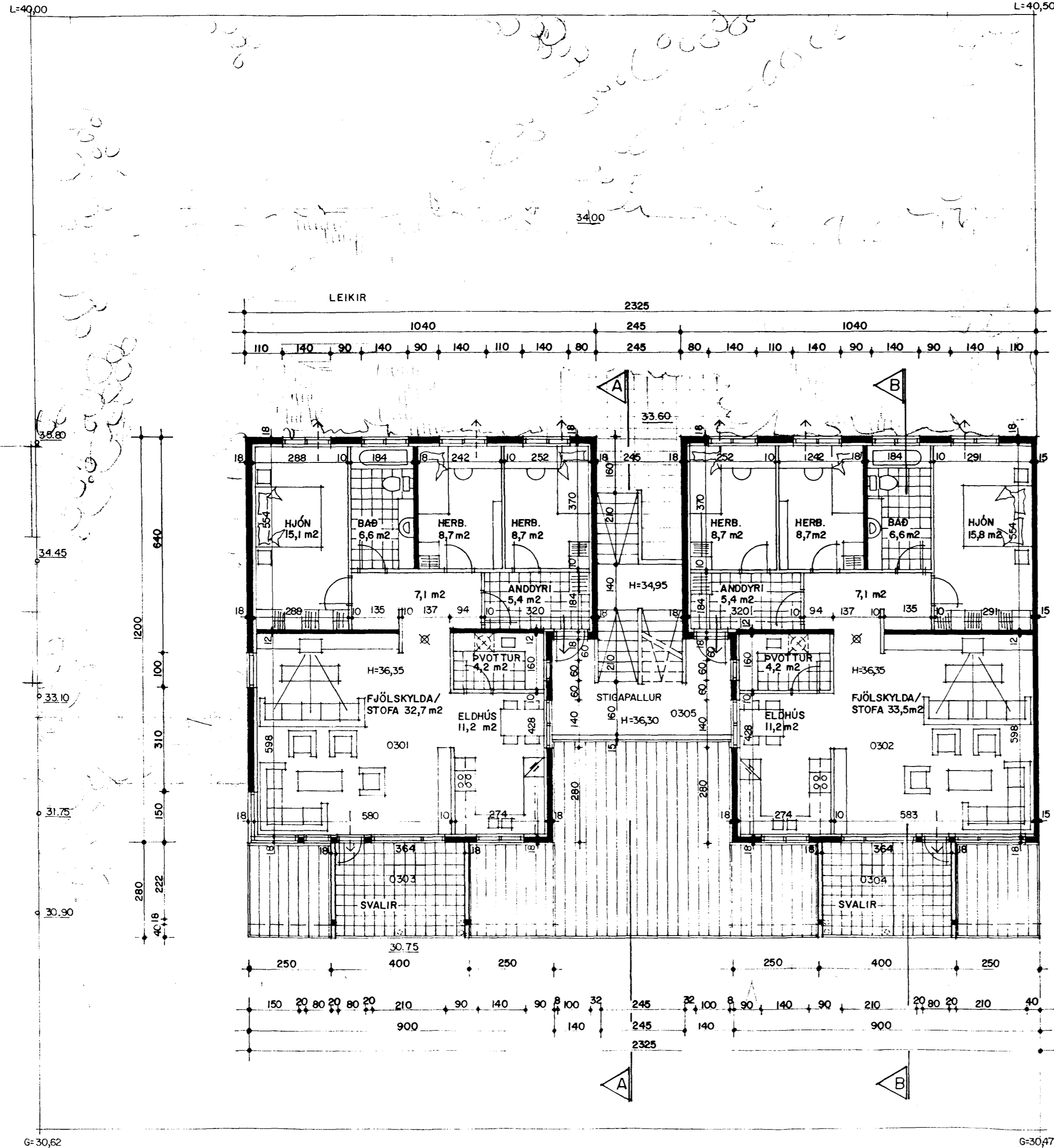
GRUNNMYND 3 HÆÐ MKV. 1:100.
