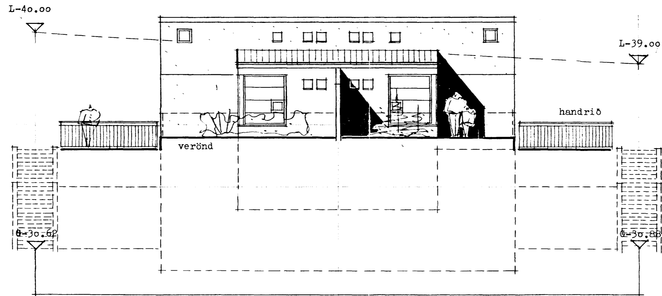
útlit norð-austur 1:100
