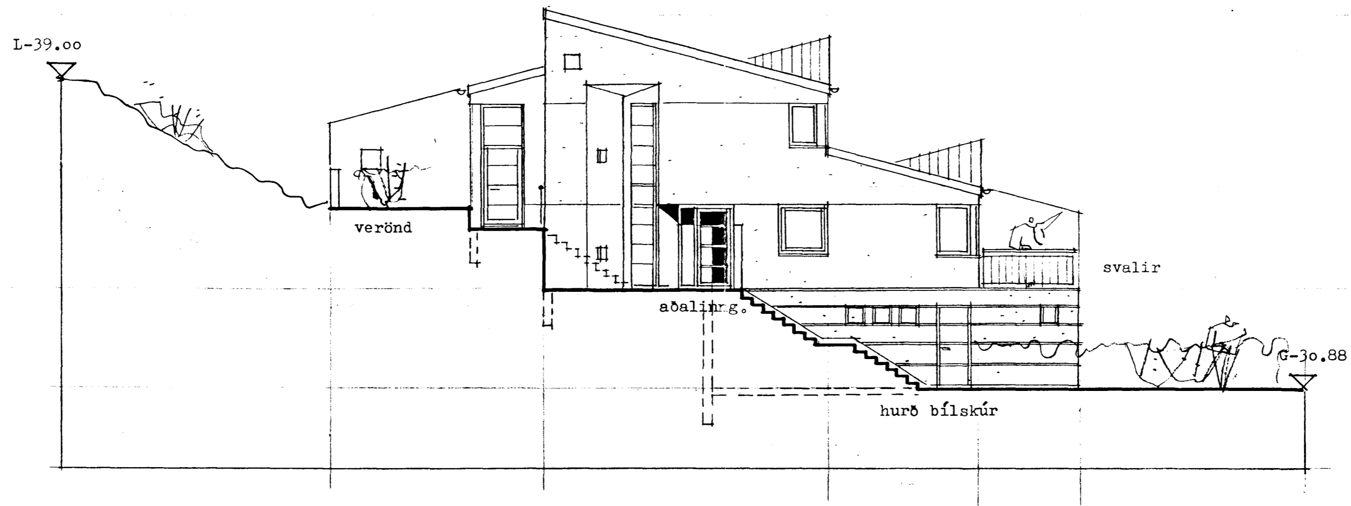
útlit norð-vestur 1:100
