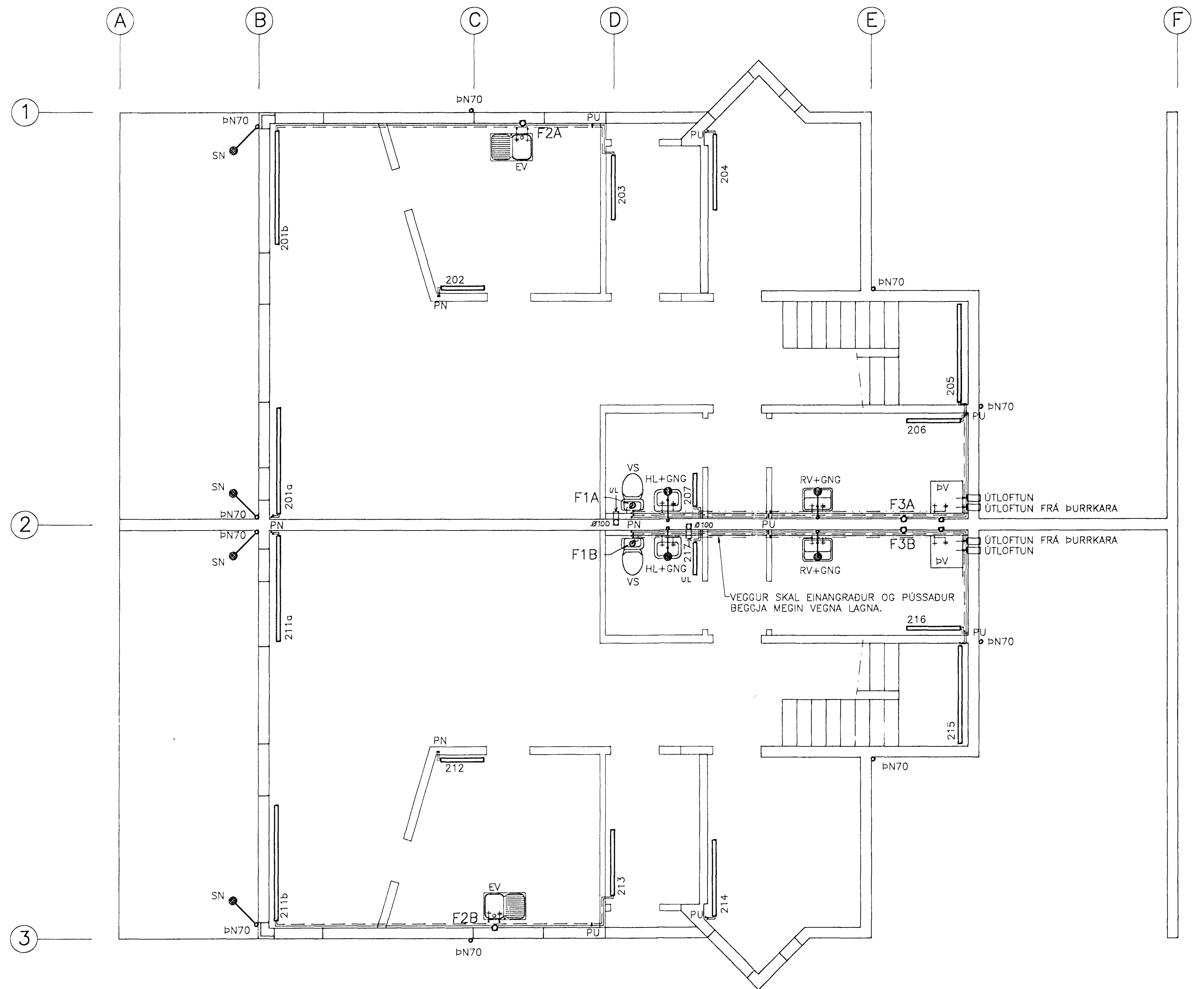
GRUNNMYND 2.HÆÐAR 1:50
