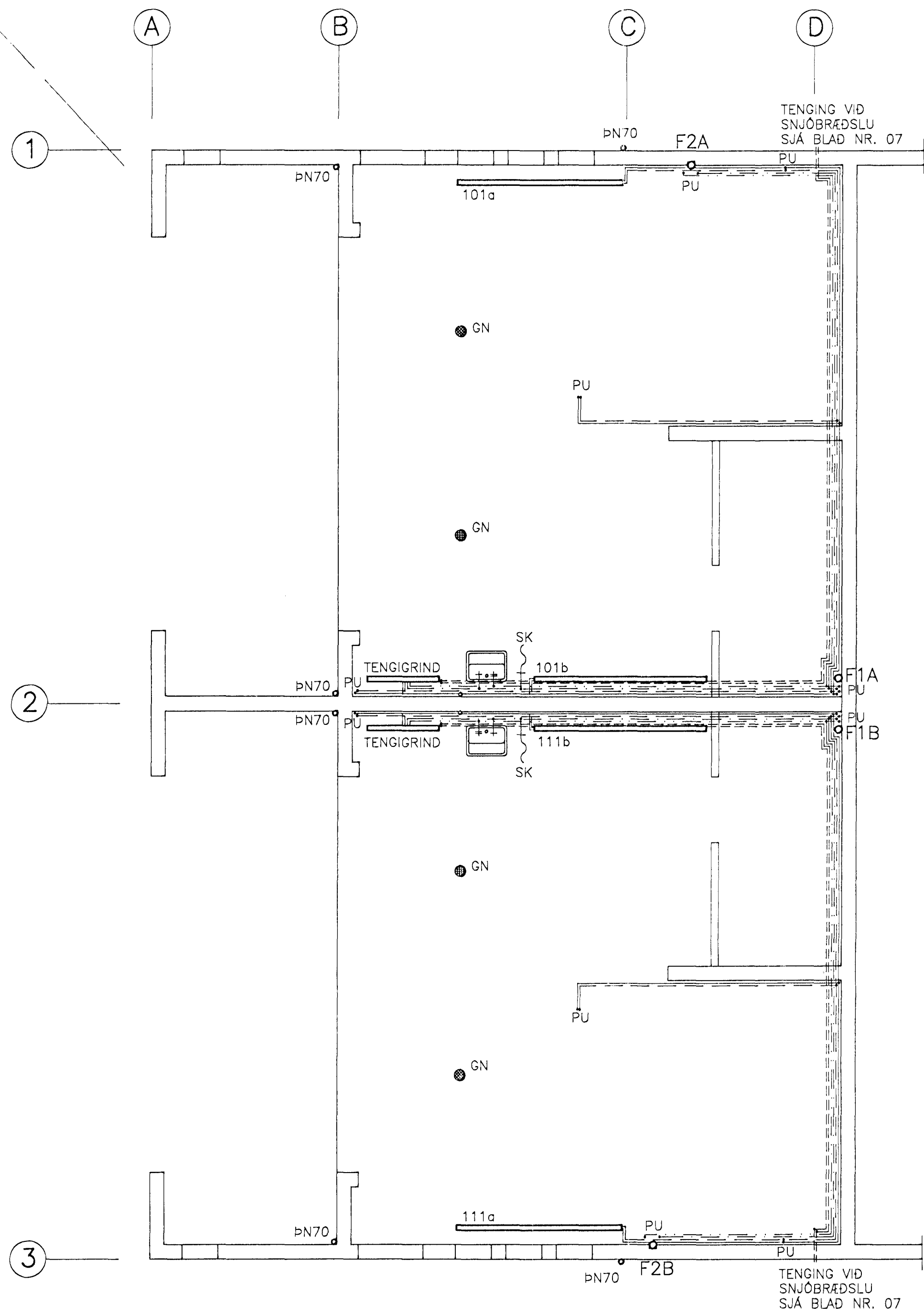
GRUNNMYND 1.HÆÐAR 1:50
