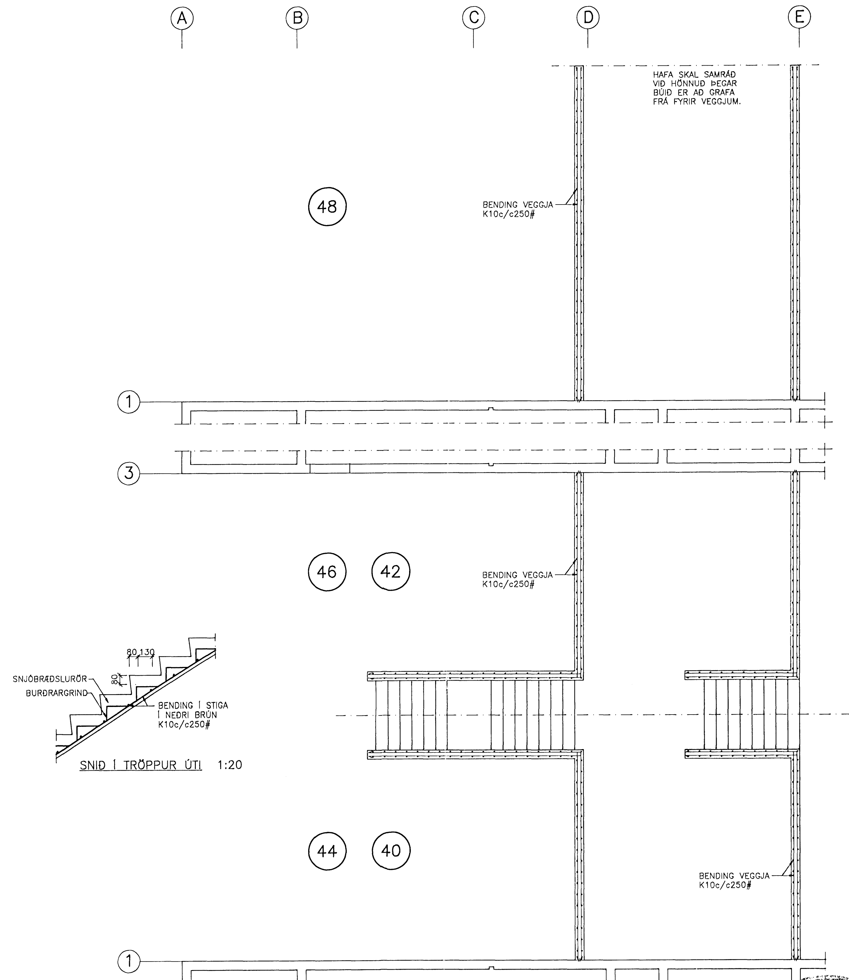
TRÖPPUR OG VEGGIR Á LÖÐ 1:50
