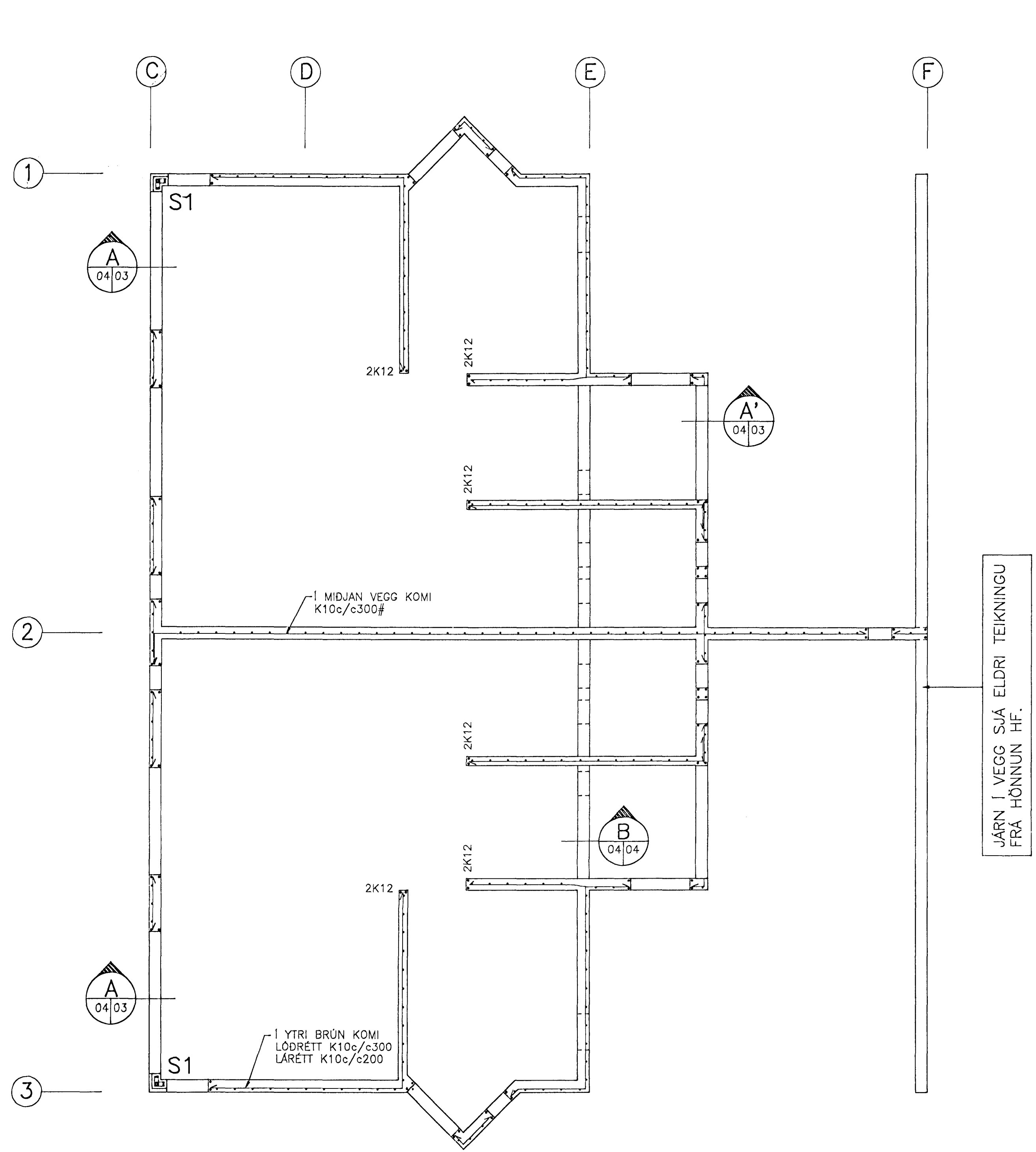
GRUNNMYND 3. HÆÐAR 1:50
