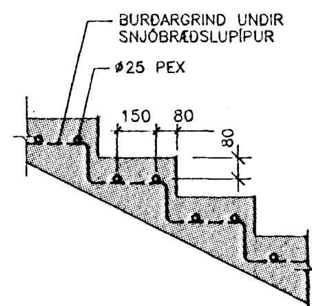
SNID I TRÖPPUR. 1:20
