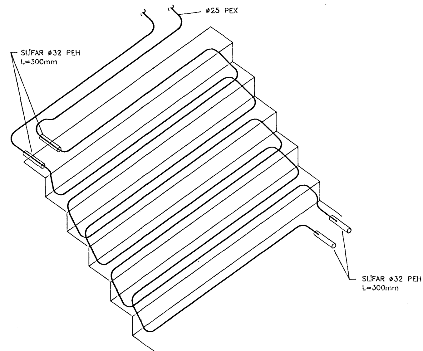
SNJÖBRÆDSLULÖGN I TRÖPPUM 1:20
