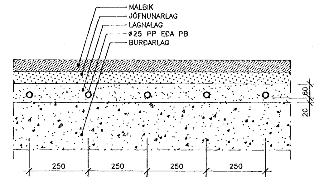
SNID I SNJÖBRÆDSLULÖGN UNDIR MALBIKI. 1:10
