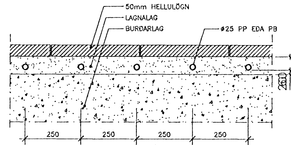
SNID I SNJÖBRÆDSLULÖGN UNDIR HELLUM. 1:10
