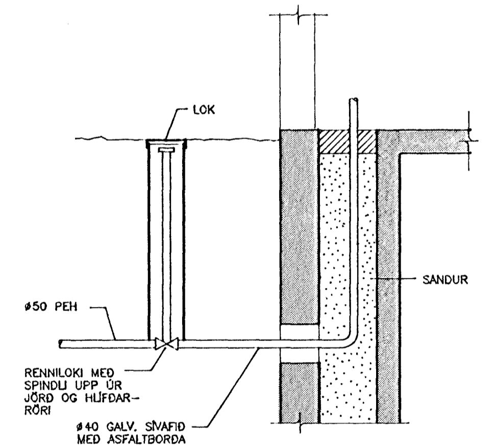
INNTAK FYRIR NEYSLUVATN, 1:20
