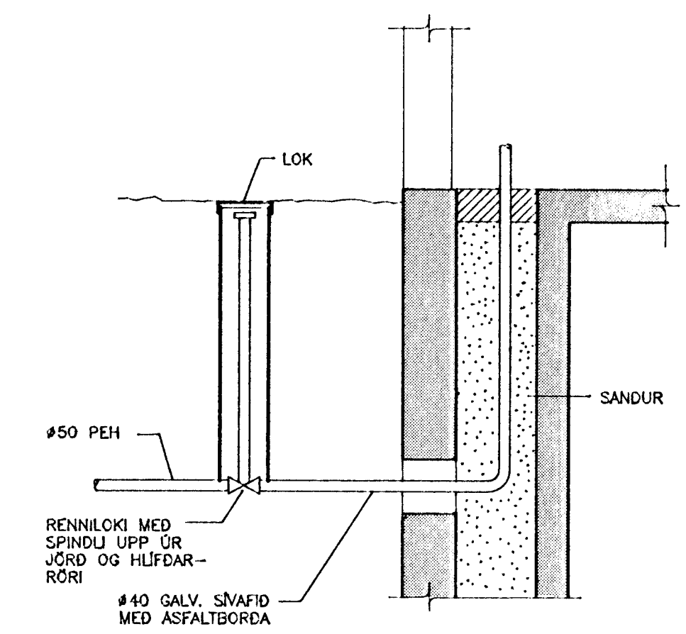
INNIÁK FYRIR NEYSLVATN, 1:20
