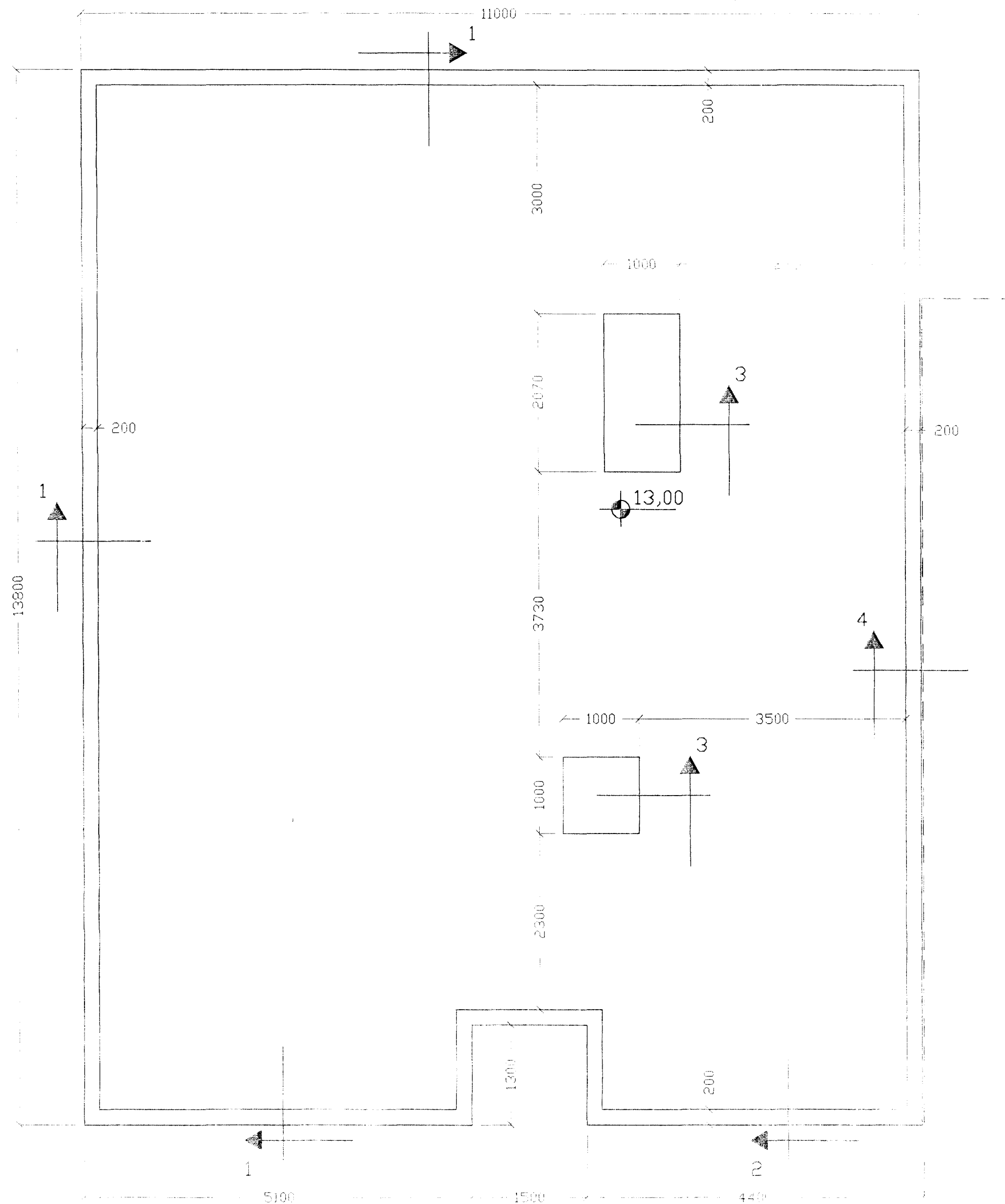
Grindmynd 1:50
