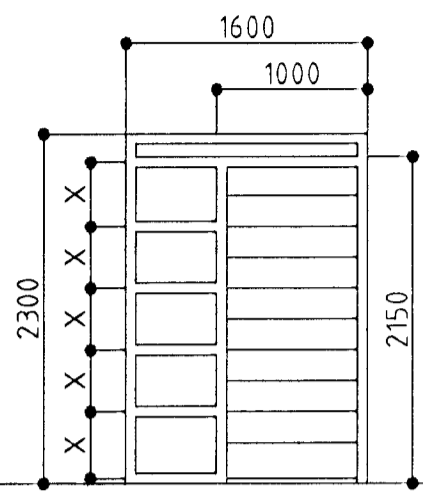
1 STK. ANDDYRI. HURÐ OPNAST HÆGRI ÚT.
