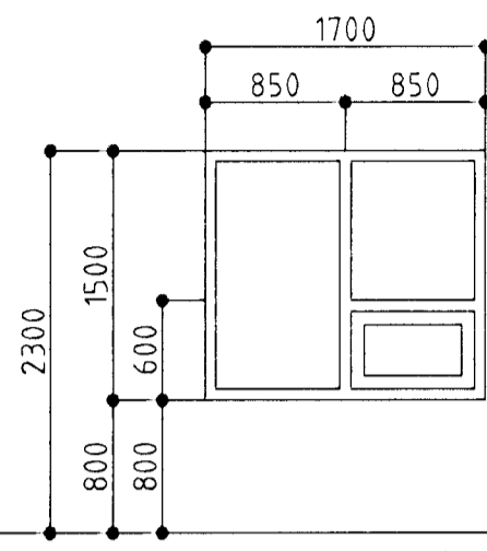
2 STK. SVEFNHERB. / HERB.
