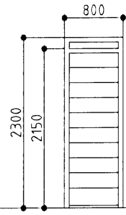
1 STK. BÍLGEYMSLA. HURÐ OPNAST HÆGRI INN.
