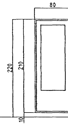
1 STK. ELDHÚS/STOFA. HURÐ OPNAST VINSTRI ÚT.
