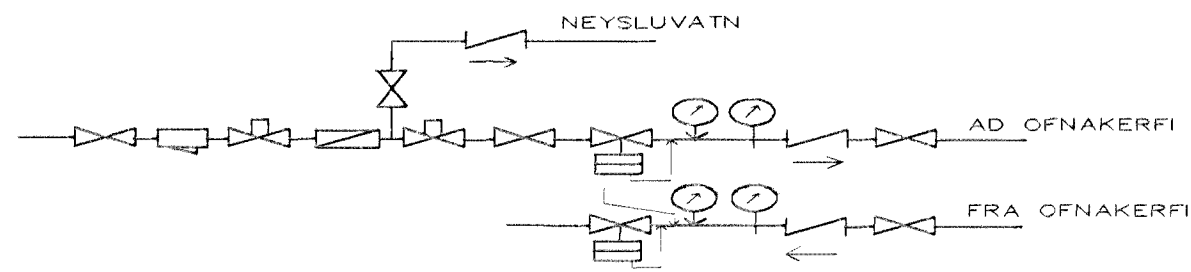
MÆLAGRIND HITAVEITU
