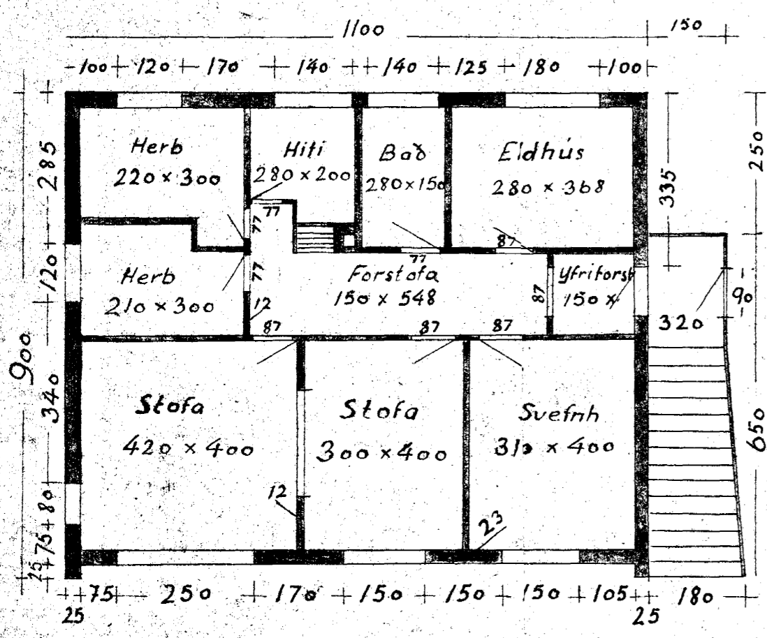
I. hæð
