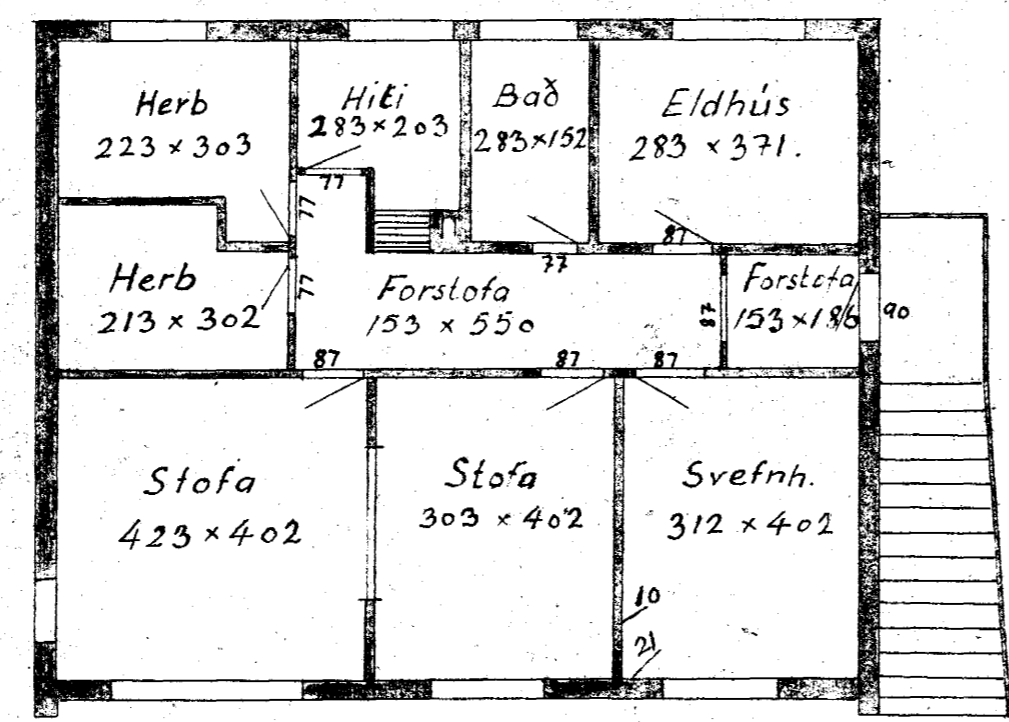
II. hæð
