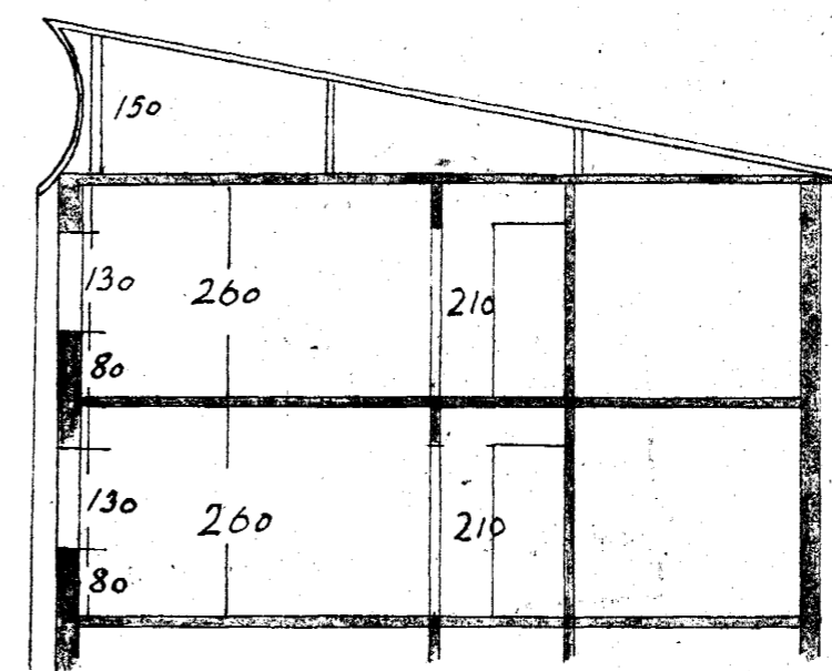
Snid A-A
