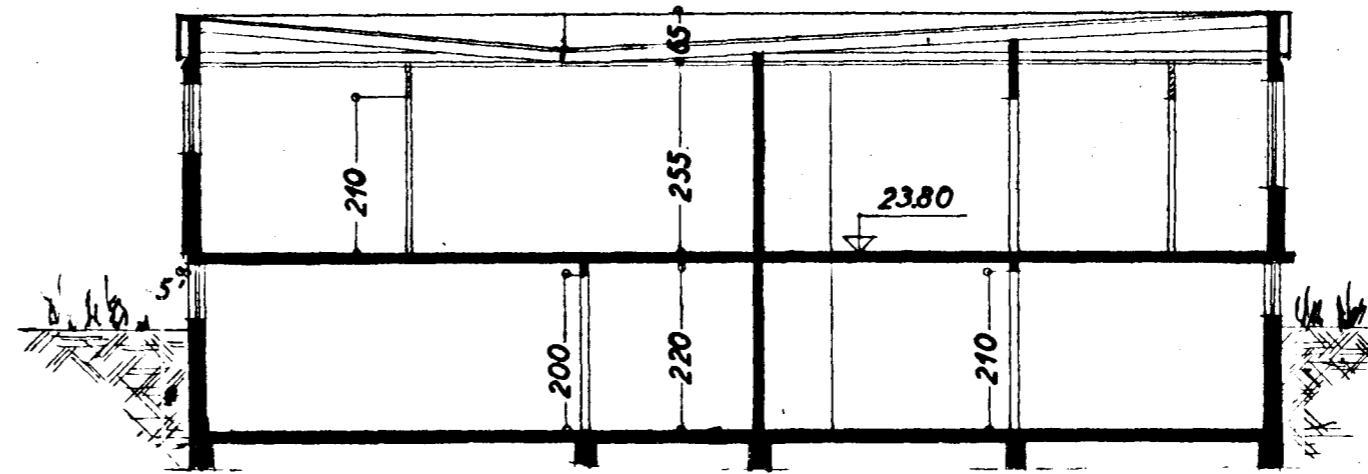
Snið: A-A
