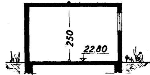
Snið: B-B
