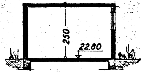
Snið: B-B
