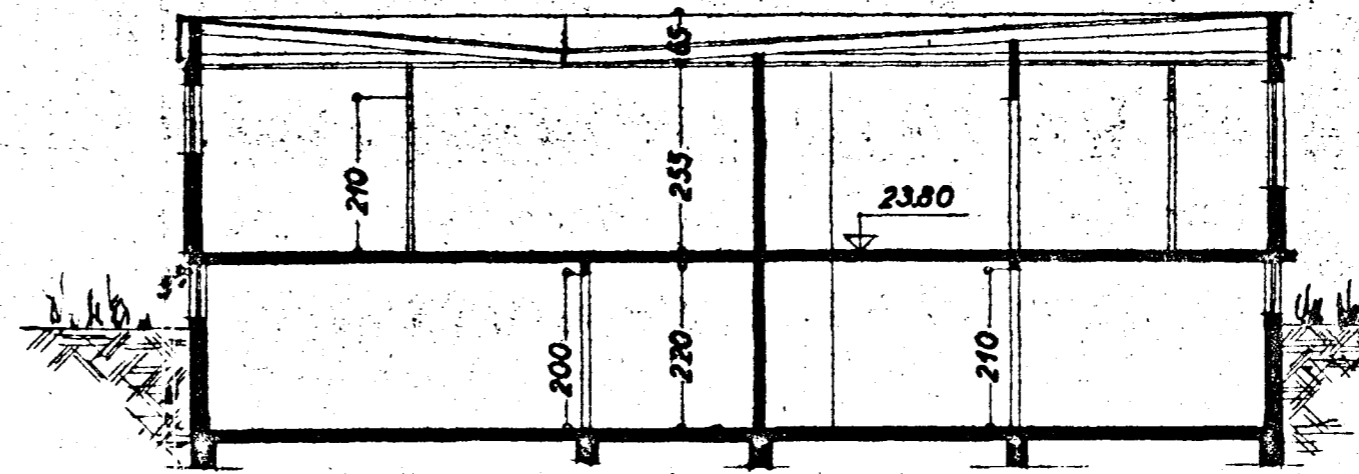
Snið: A-A
