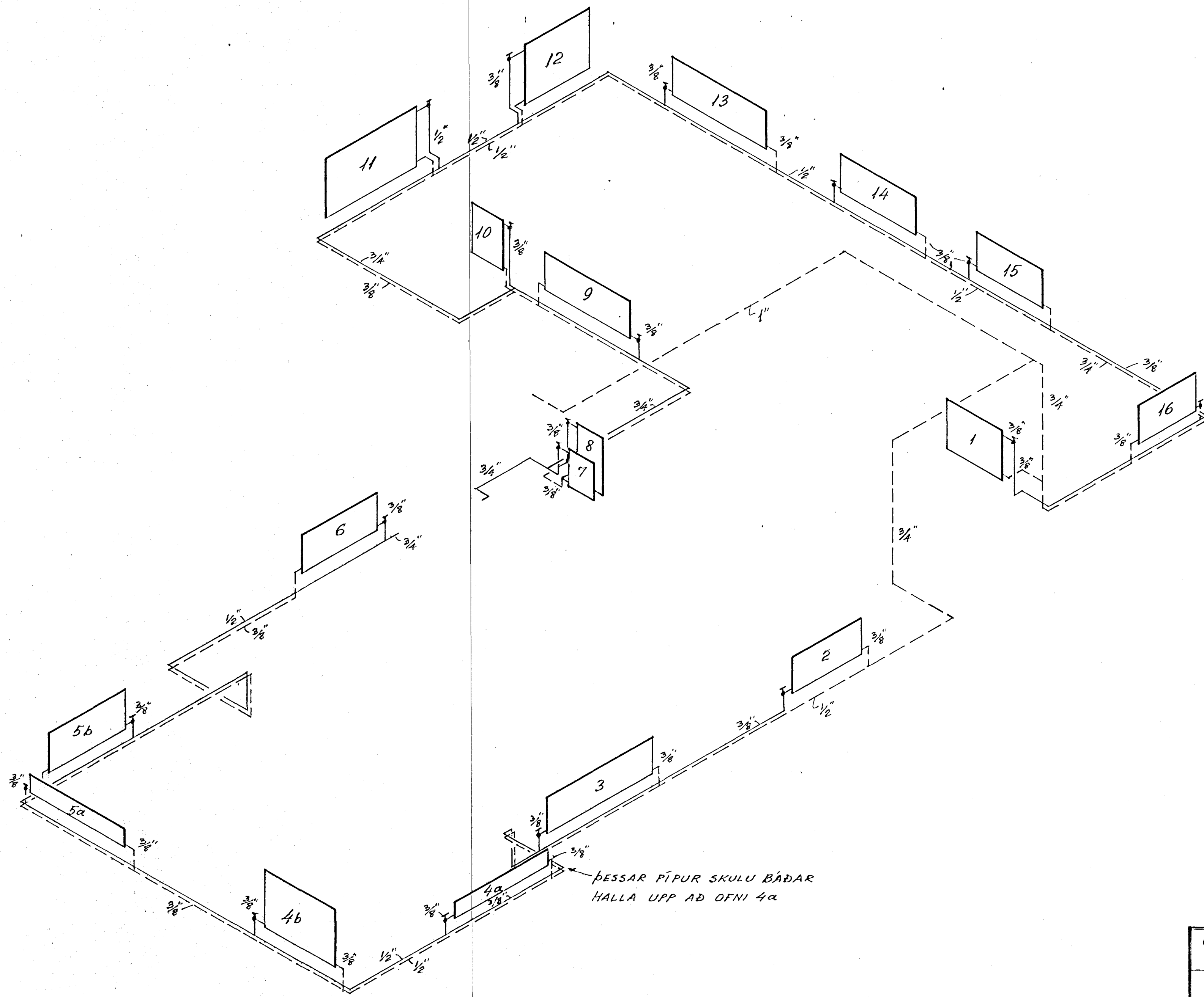
PÍPUKERFI 1:50
