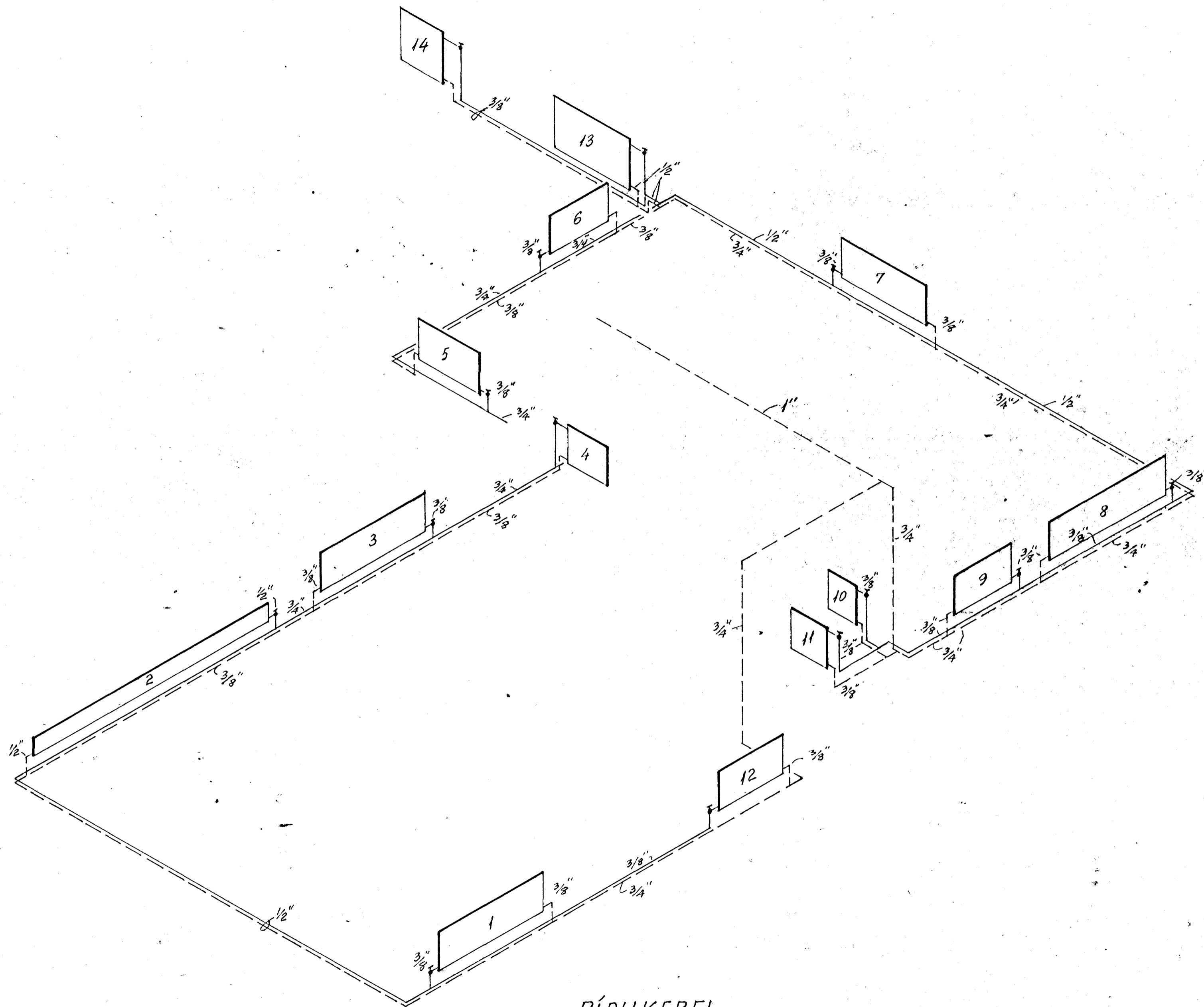
PÍPUKERFI 1:50
