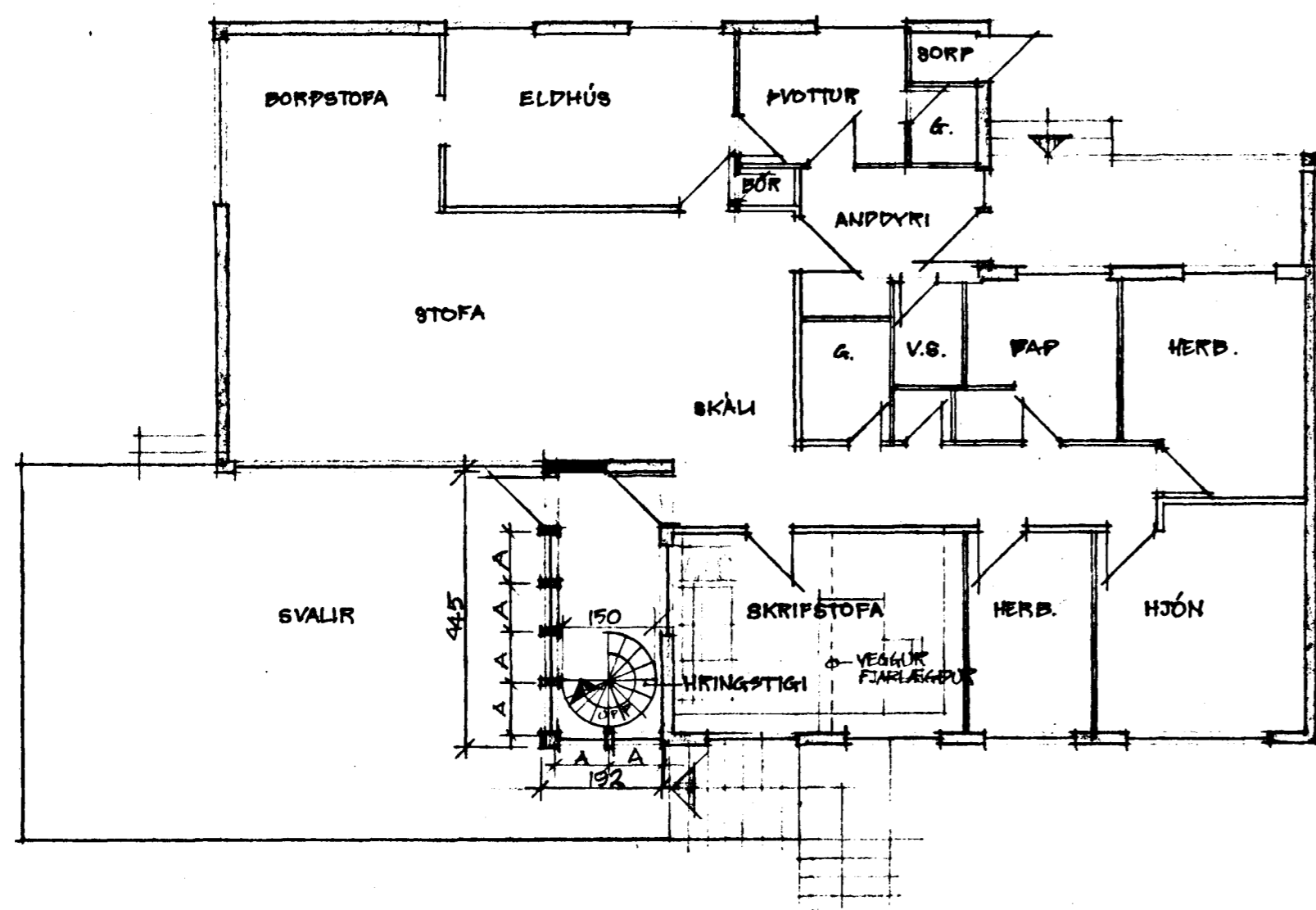
GRUNNMYND JARÐHEÐAR
