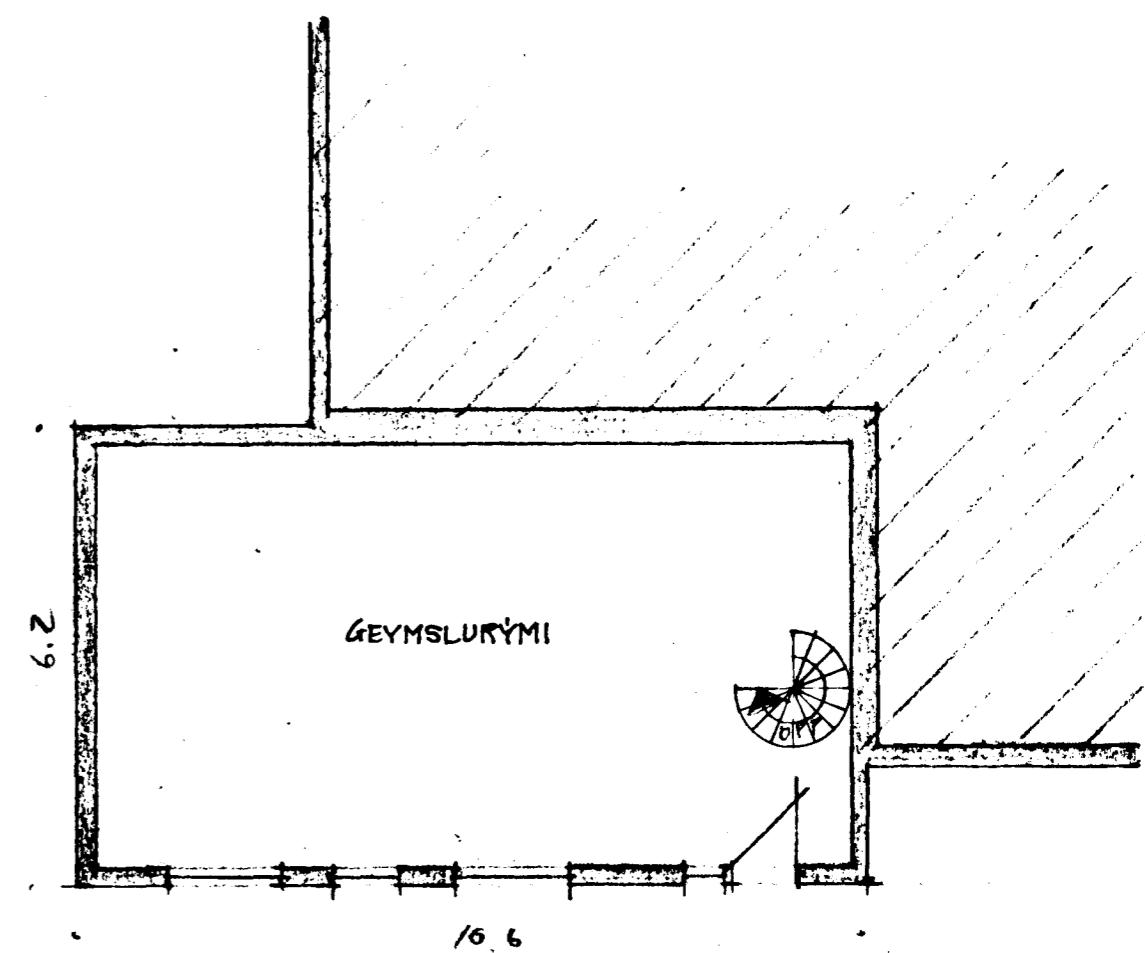
GRUNNMYND KJALLARA
