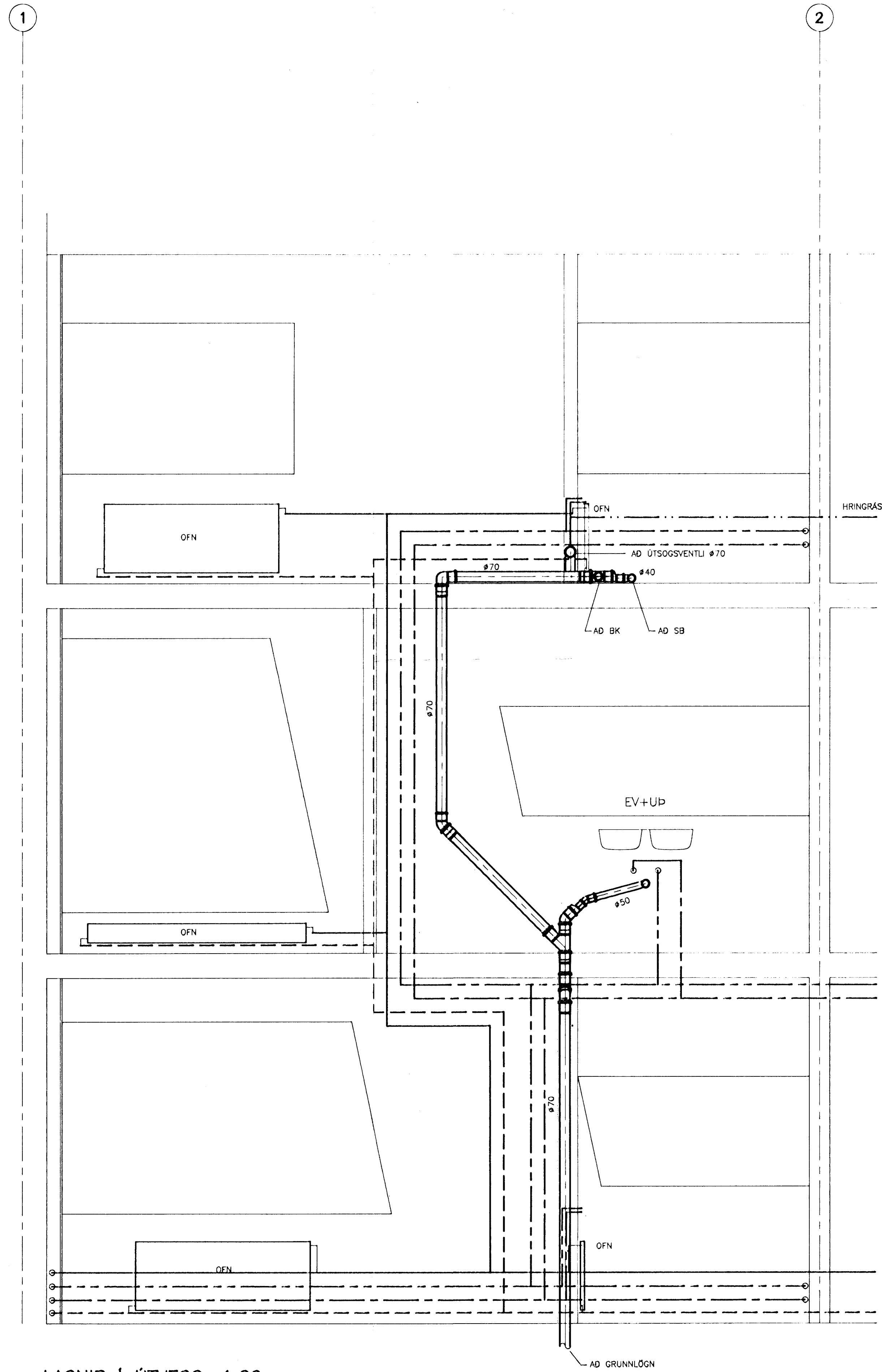
LAGNIR I ÚTVEGG, 1:20
