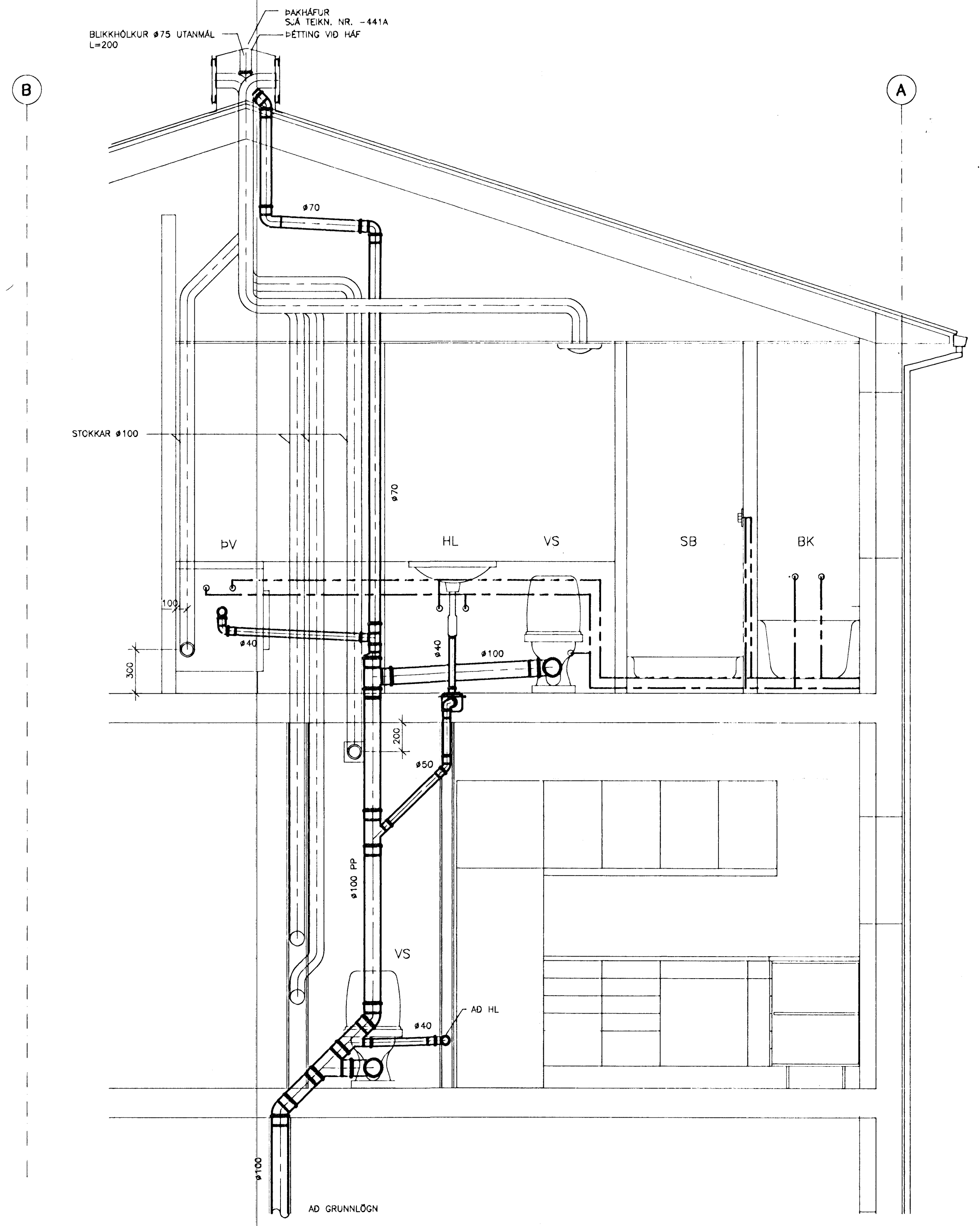
LAGNIR I LAGNAVEGGJUM, 1:20
