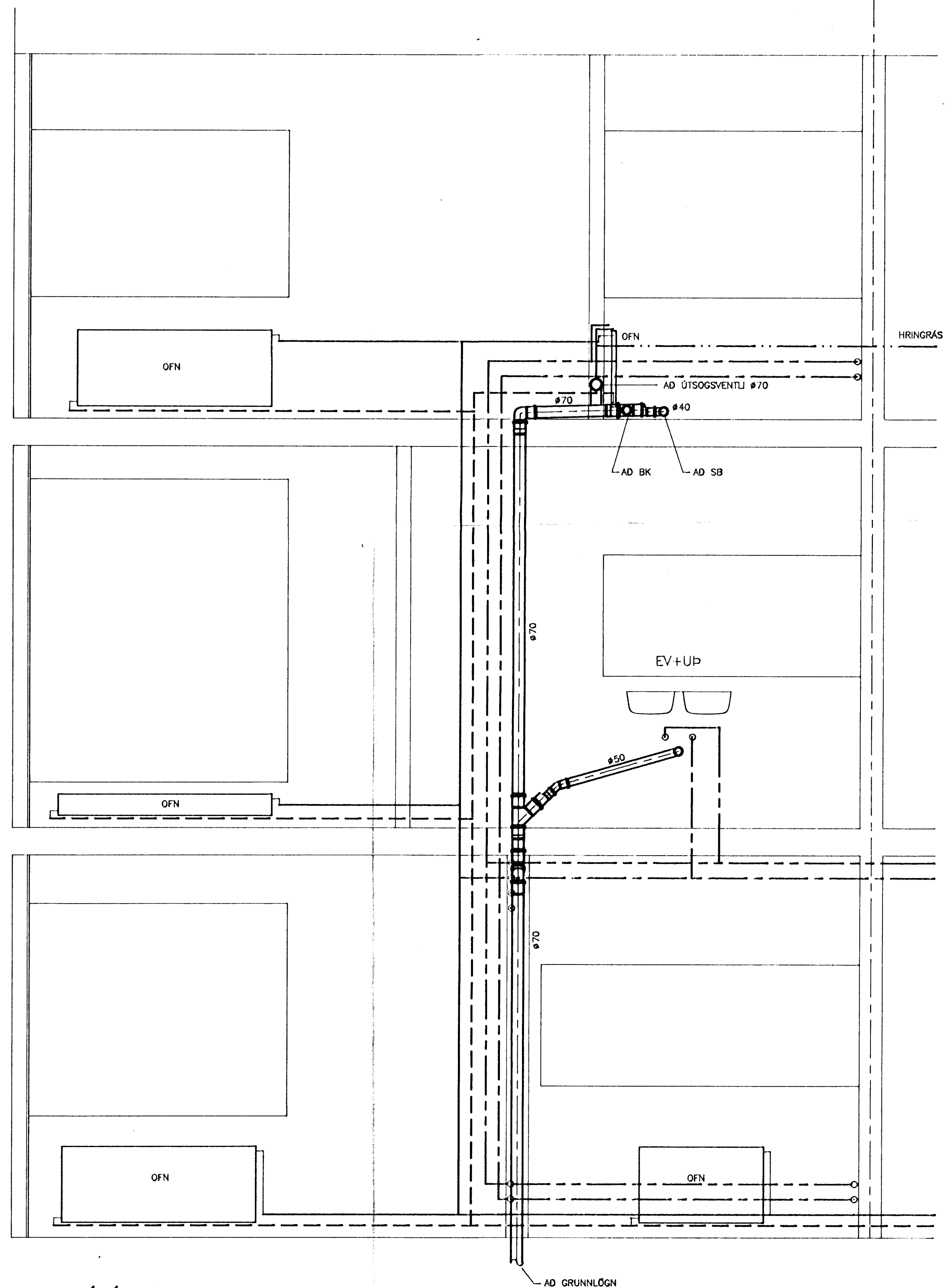
LAGNIR Í ÚTVEGG, 1:20
