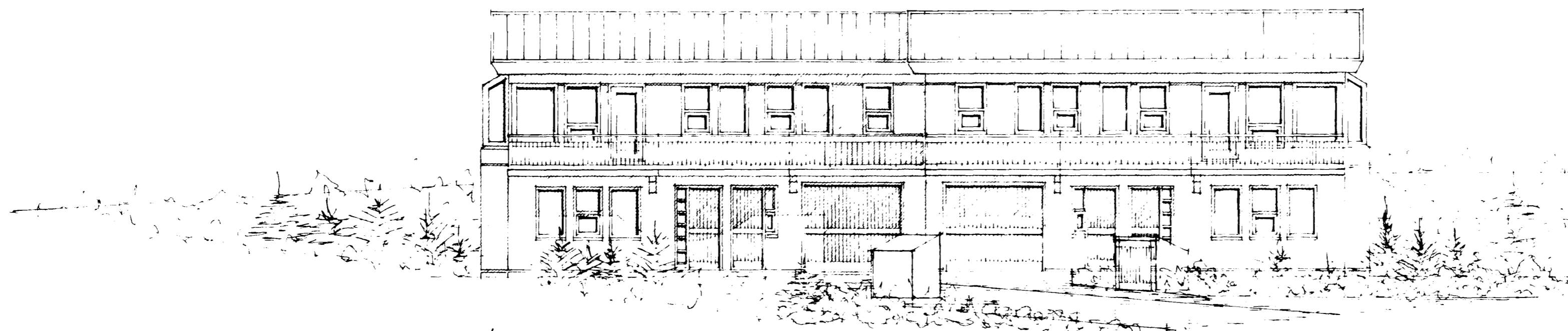
ÚTLIT SUÐVESTUR MKV. 1:100.
