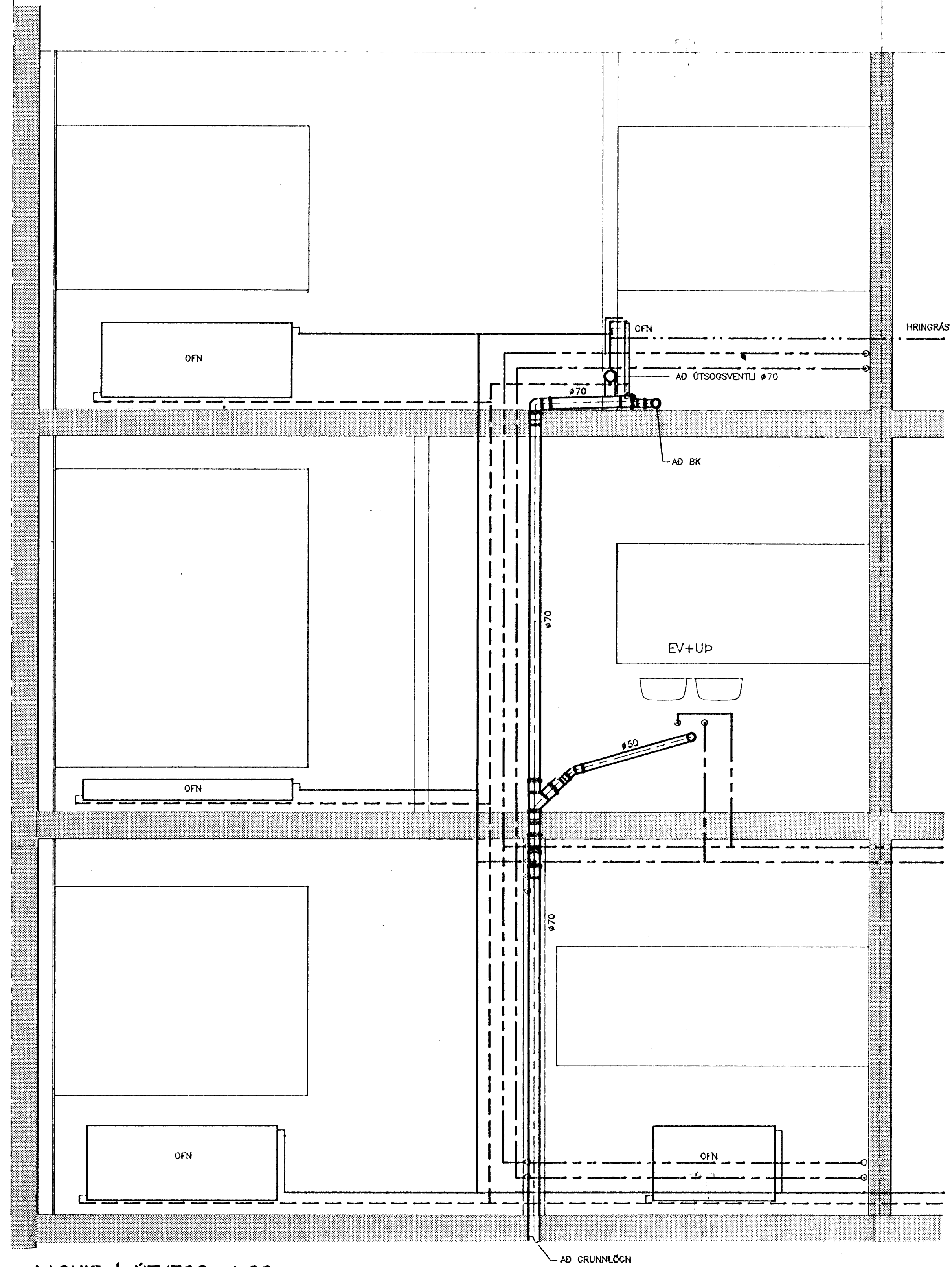
LAGNIR I ÚTVEGG, 1:20
