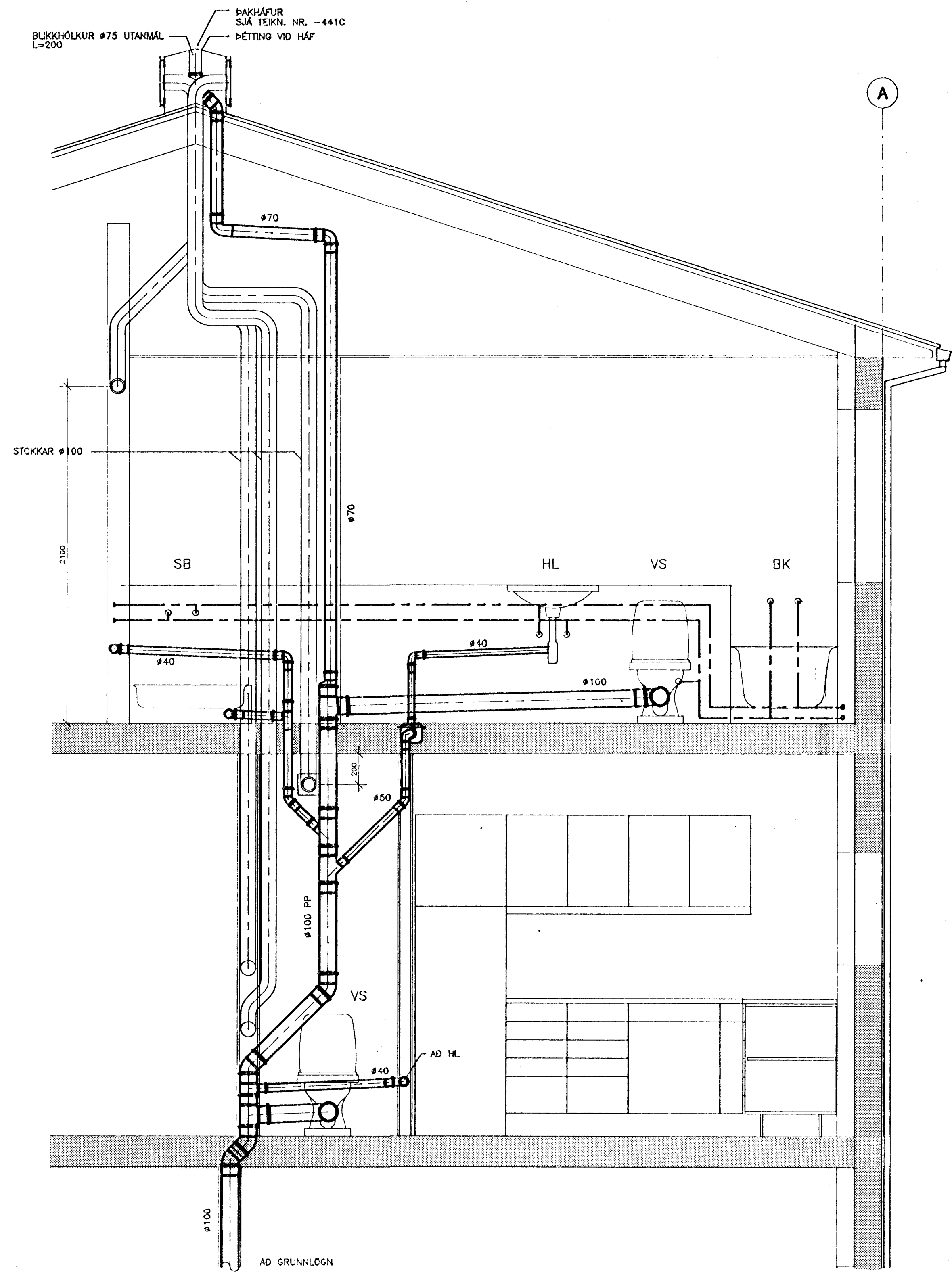
LAGNIR I LAGNAVEGGJUM, 1:20
